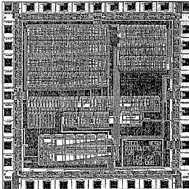
IC LAYOUT
