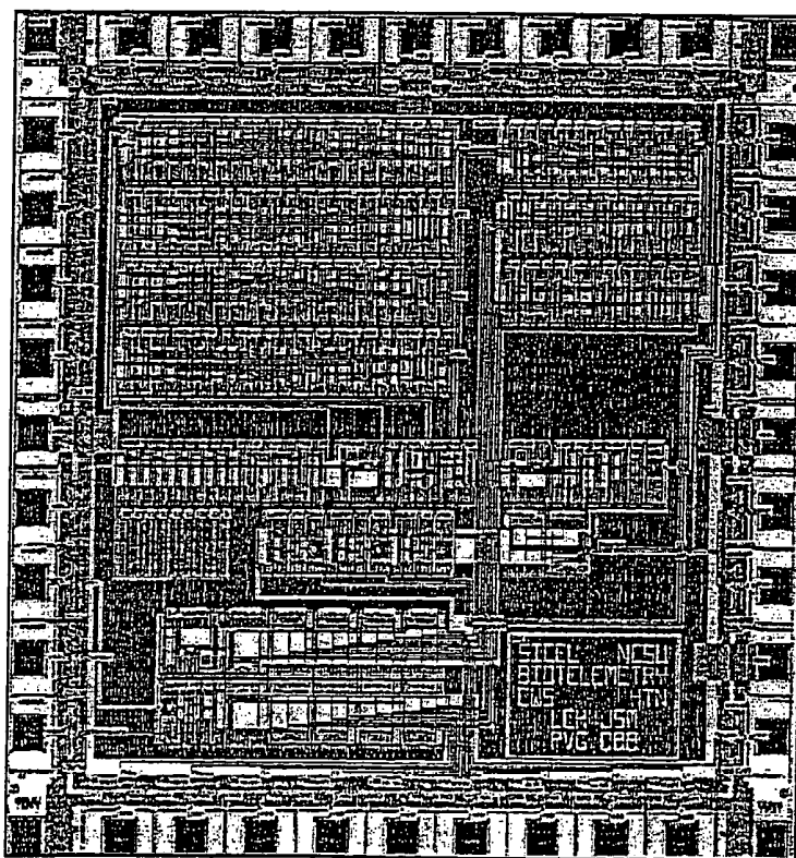
IC LAYOUT
