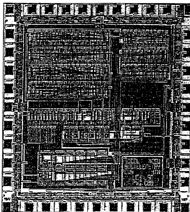
IC LAYOUT
