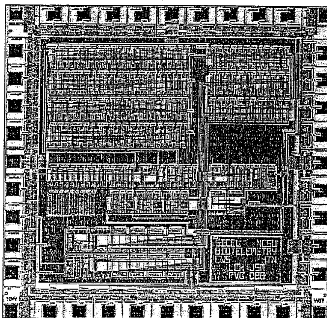
IC LAYOUT
