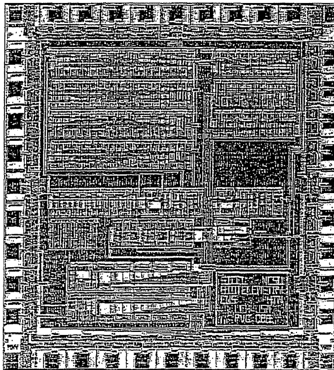
IC LAYOUT
