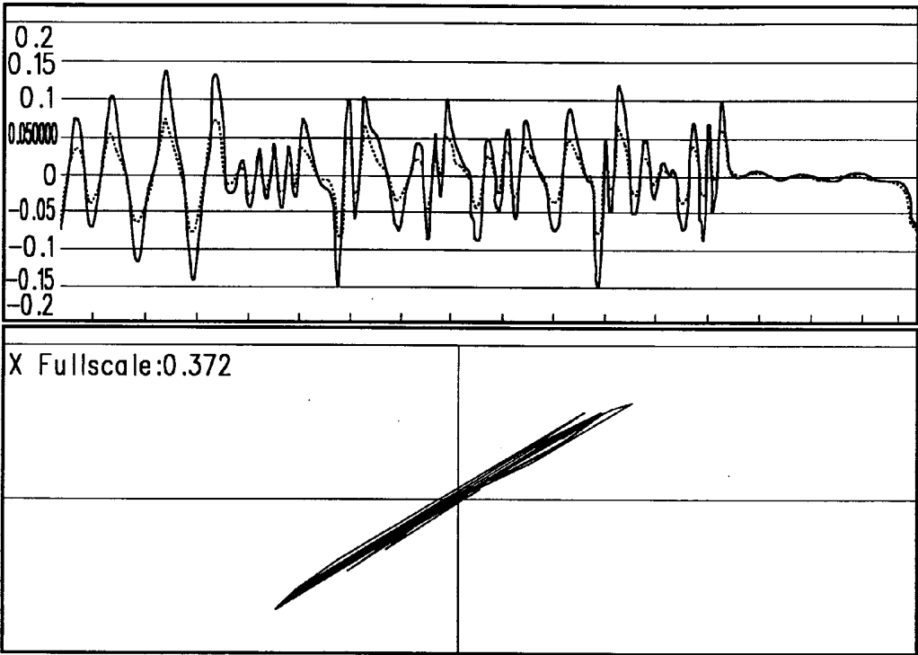
FIG. 11B
