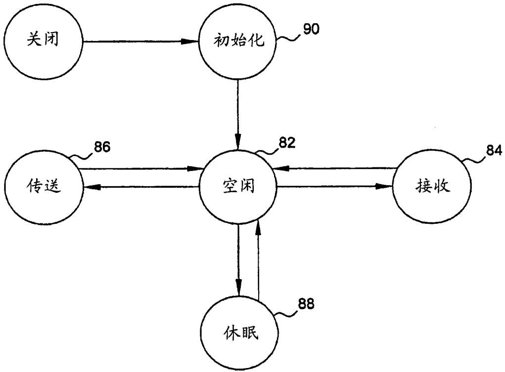
无线电模块状态转移图
