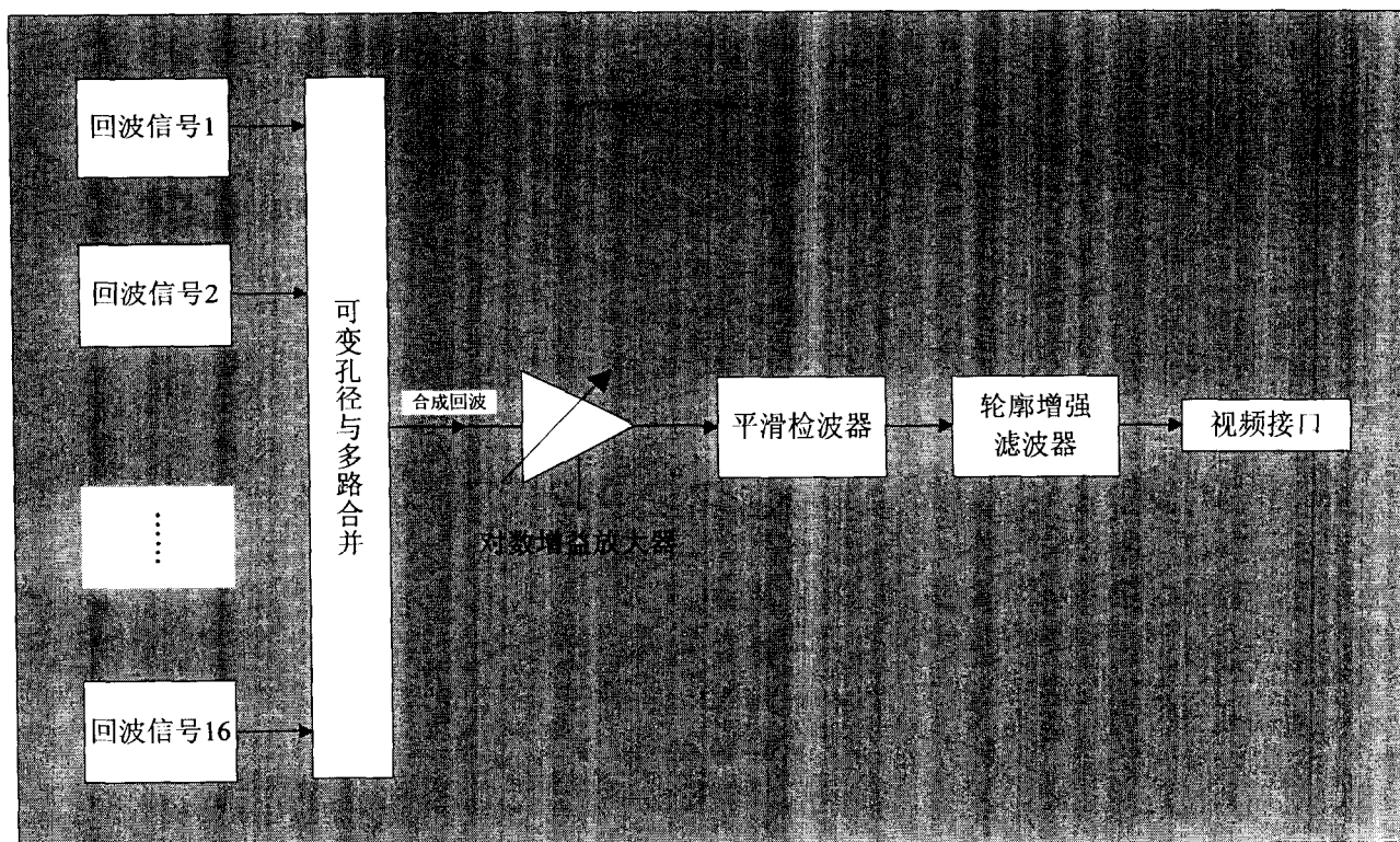
图 11 超声回波合成与后处理
