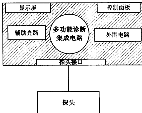
图 1 多功能医疗诊断设备基本结构图
