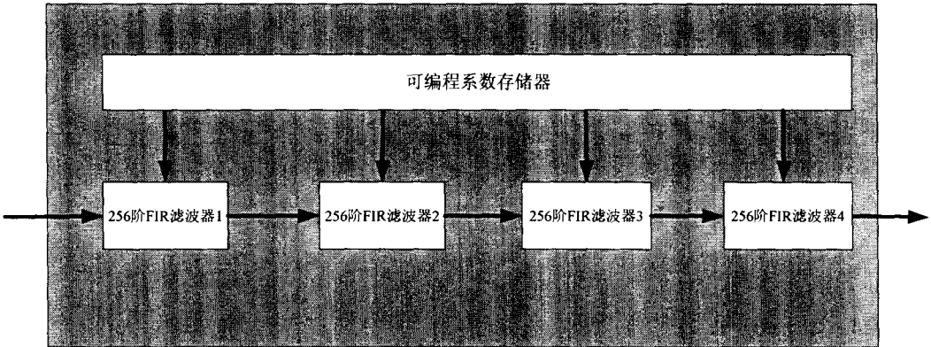
图 7 可编程通道滤波器
