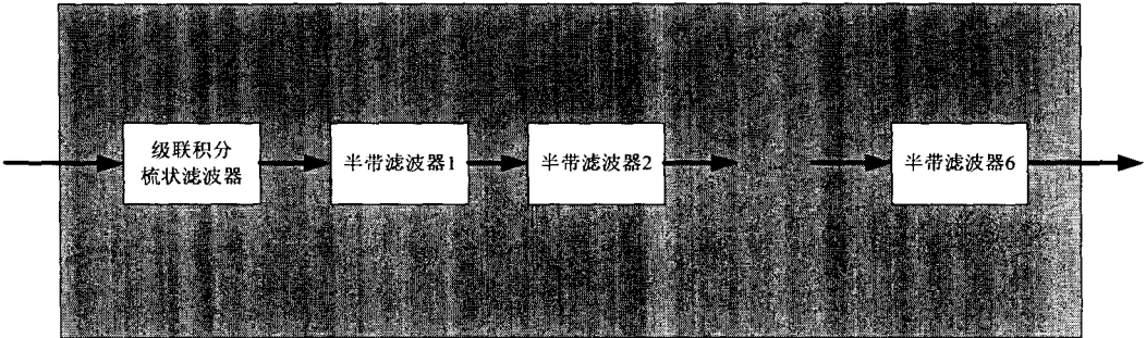
图 6 可编程采样率抽取
