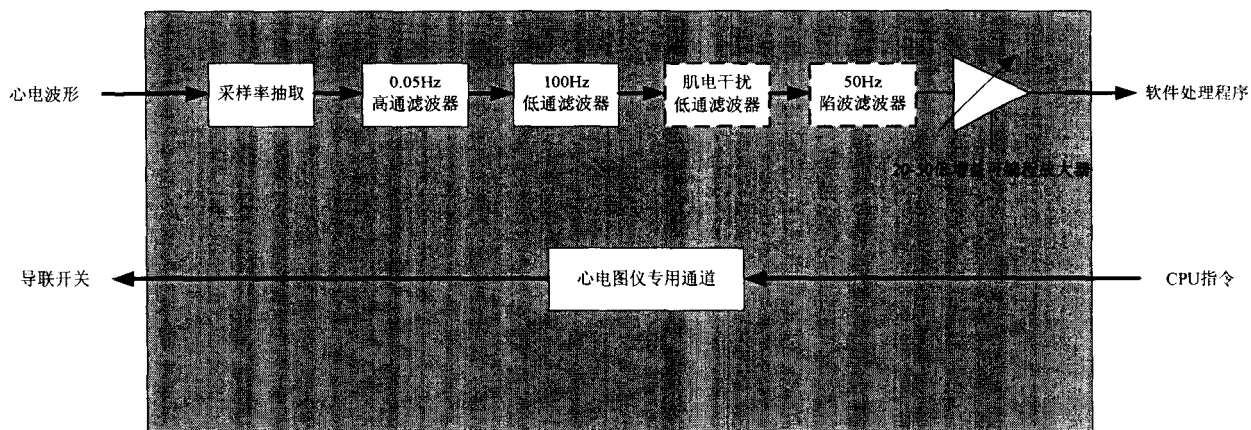
图 9 心电图模式后续处理模块
