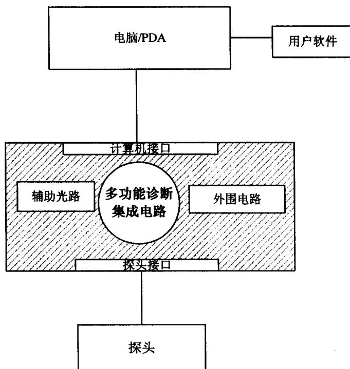
图 2 外接计算机的多功能医疗诊断设备结构图
