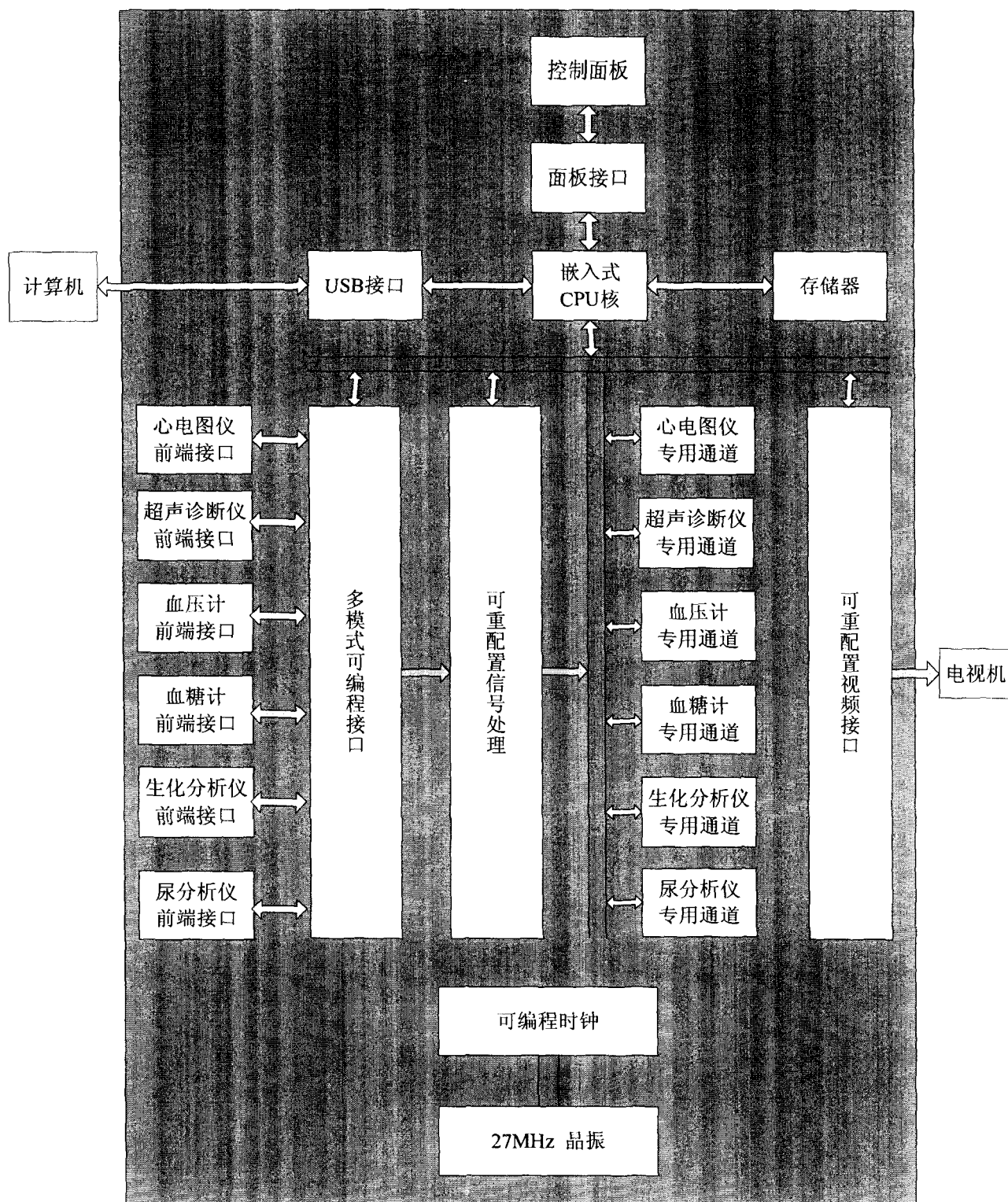
图4 多功能诊断设备电路总体结构图
