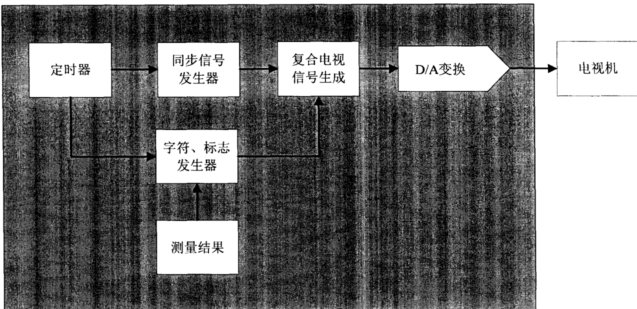
图 15 心电图模式视频接口
