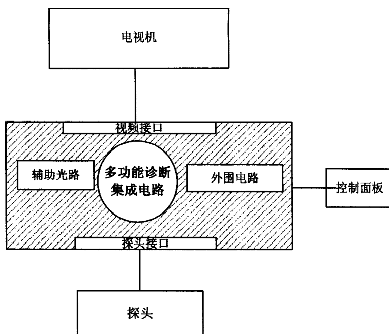
图3 外接电视机的多功能医疗诊断设备结构图
