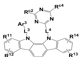
[화학식 B-ET-a]
