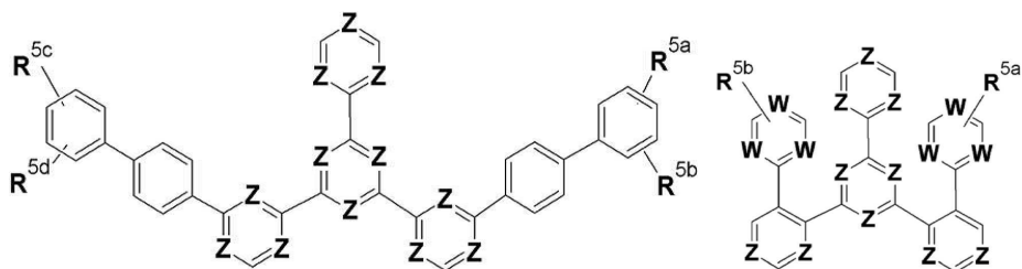
[화학식 1-VIII]
