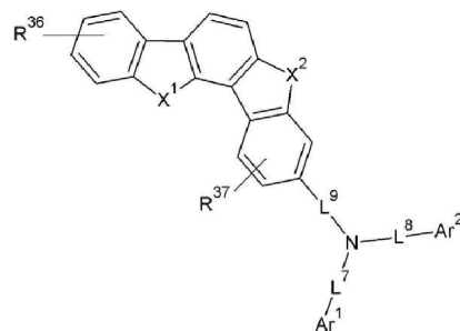
[화학식 2-2]
