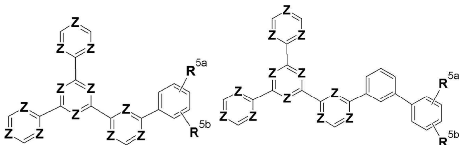
[화학식 1-V]
