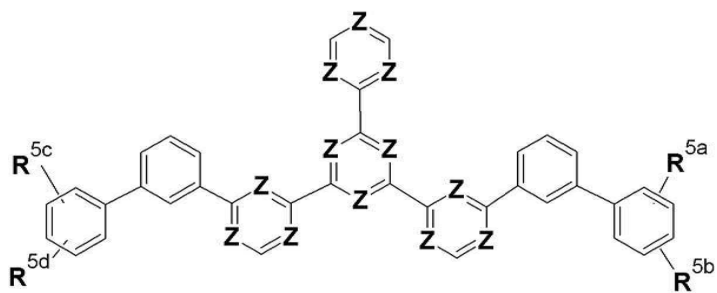
[화학식 1-VIII]
