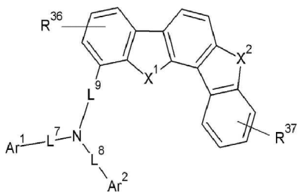
[화학식 2-1]
