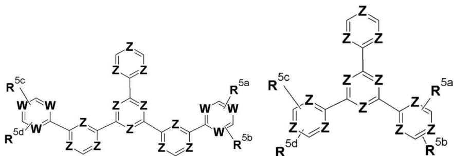
[화학식 1-VII]
