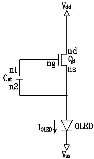
도면7
