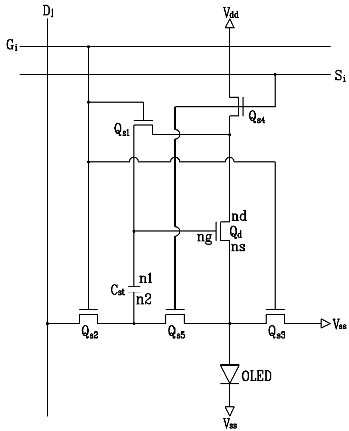
도면2
