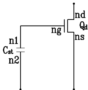
도면6c
