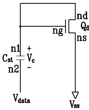
도면6c
