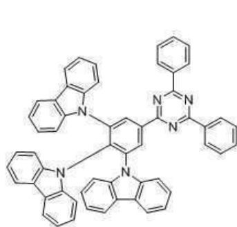
화합물 1
