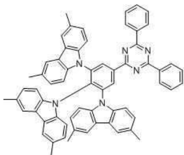
화합물 2
