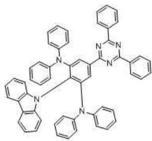
화합물 7
