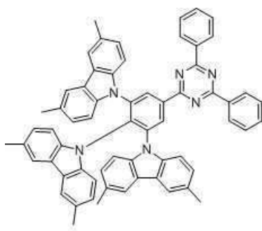
화합물 2
