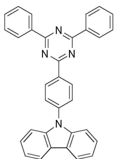
<화합물 8>
