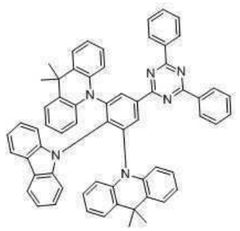
화합물 3
