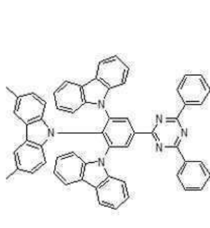
화합물 6
