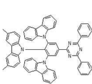
화합물 6
