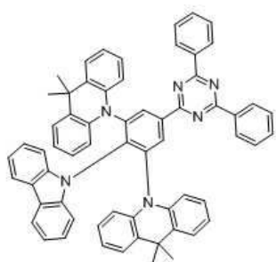
화합물 3
