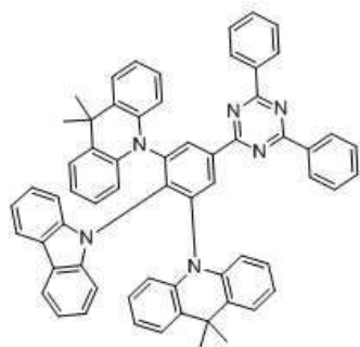
화합물 3
