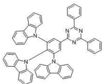
화합물 1
