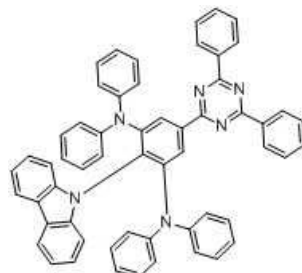
화합물 7
