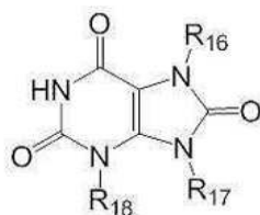
[화학식 3g]
