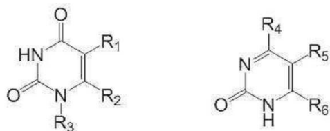
[화학식 3a]
