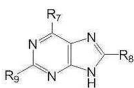
[화학식 3c]
