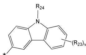
화학식 4E
