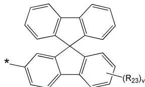
화학식 4D
