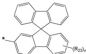
화학식 4D
