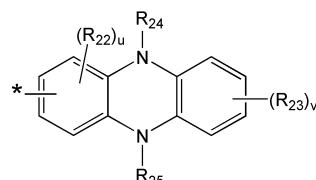
화학식 3R
