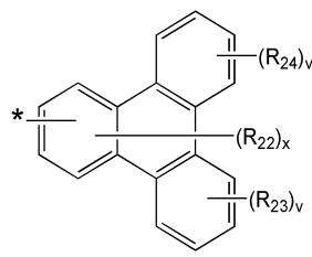
화학식 3I
