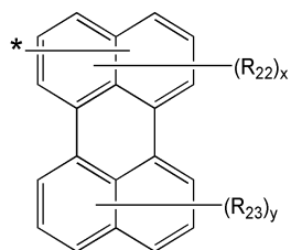
화학식 3J
