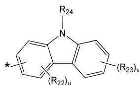
화학식 3E
