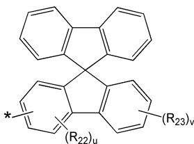
화학식 3D
