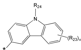
화학식 4E
