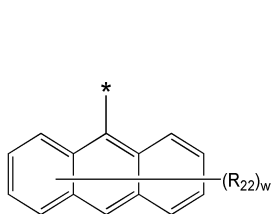
화학식 4G
