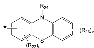
화학식 3Q
