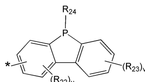
화학식 3O
