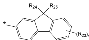
화학식 4C
