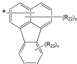
화학식 3K
