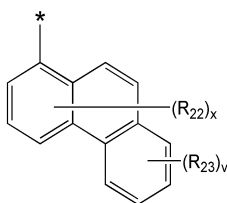
화학식 4H
