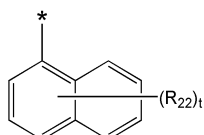
화학식 4B
