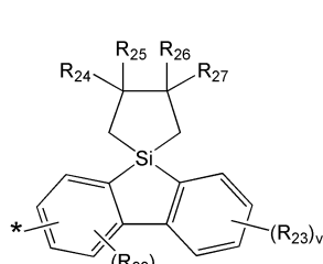
화학식 3M
