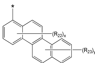
화학식 4I
