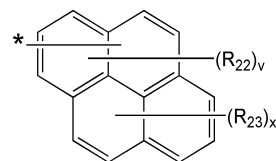
화학식 3L
