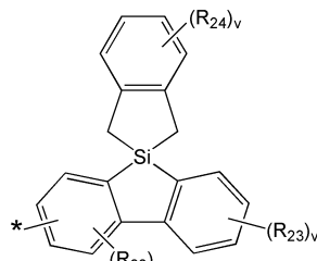
화학식 3N
