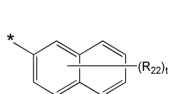
화학식 4A
