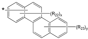
화학식 3H
