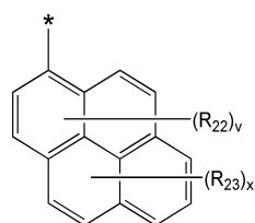
화학식 4J
