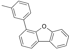
화학식 (Ar-17a3)
