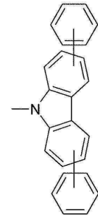
화학식 (Ar1-15)
