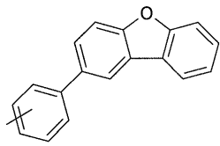
화학식 (Ar-17c)
