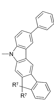
화학식 (Ar1-17a)
