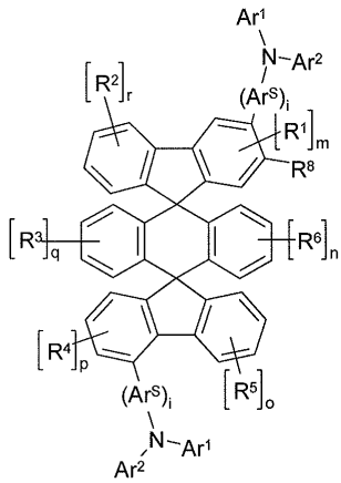
화학식 (26)
