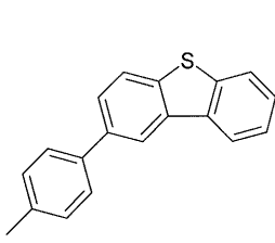
화학식 (Ar-16c1)
