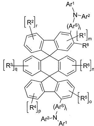
화학식 (25)
