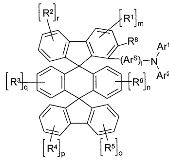
화학식 (15)
