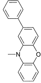
화학식 (Ar1-8b)
