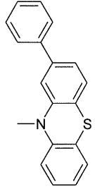
화학식 (Ar1-7b)
