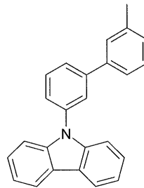
화학식 (Ar-30b)
