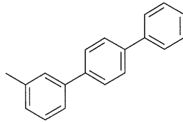
화학식 (Ar-3b)
