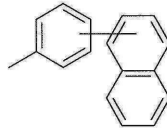
화학식 (Ar-29)
