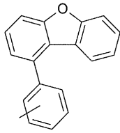
화학식 (Ar-17d)
