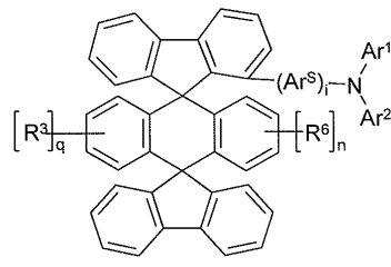
화학식 (15a)
