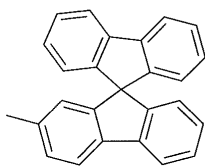
화학식 (Ar-10b)
