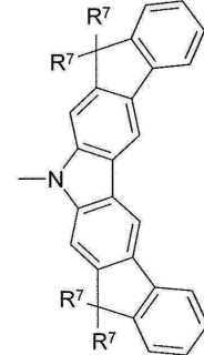
화학식 (Ar1-18)
