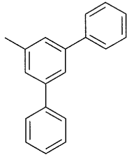
화학식 (Ar-4a)
