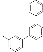
화학식 (Ar-3d)
