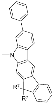
화학식 (Ar1-17b)
