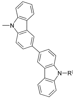
화학식 (Ar1-19)
