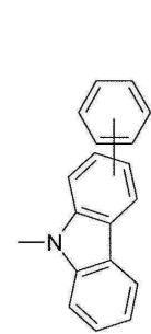
화학식 (Ar1-14)
