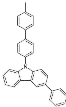
화학식 (Ar-32)
