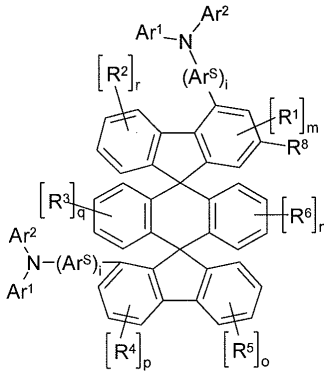
화학식 (10)
