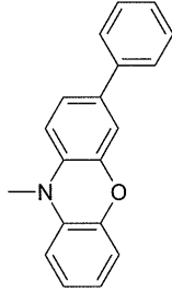
화학식 (Ar1-8a)
