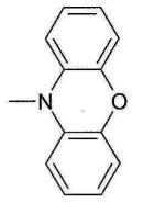
화학식 (Ar1-4)
