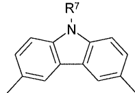
화학식 (Ar3-9a)
