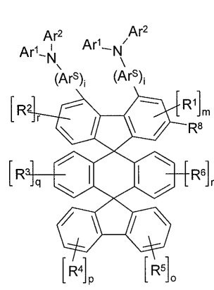
화학식 (9)
