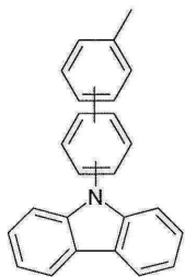
화학식 (Ar-30)
