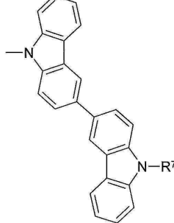
화학식 (Ar1-19)
