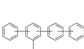
화학식 (Ar-6)
