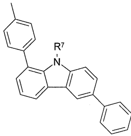
화학식 (Ar-19a)
