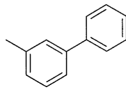
화학식 (Ar-2b)
