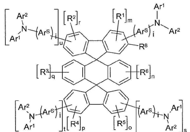
화학식 (1)
