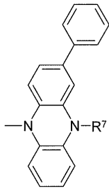
화학식 (Ar1-6a)
