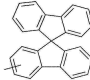
화학식 (Ar-10)
