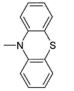
화학식 (Ar1-3)
