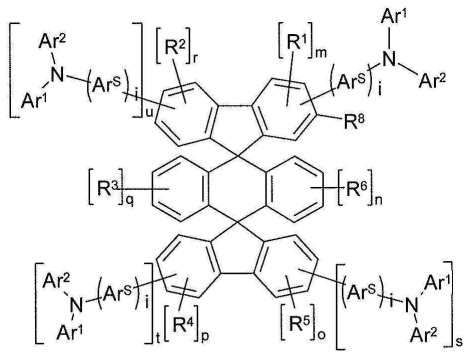
화학식 (1)
