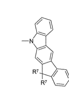
화학식 (Ar1-16)
