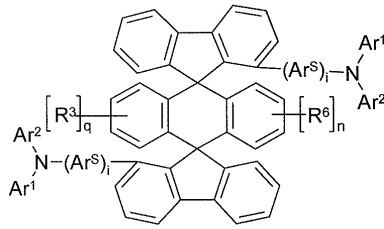
화학식 (16a)
