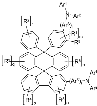
화학식 (28)
