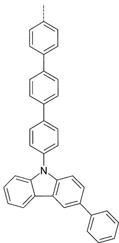
화학식 (Ar-33)
