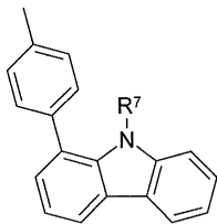
화학식 (Ar-15a1)
