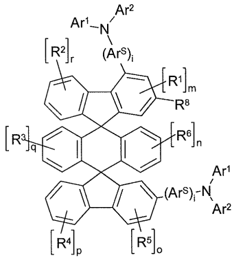
화학식 (14)
