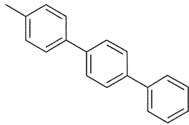
화학식 (Ar-3a)
