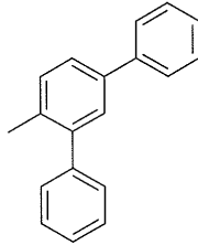
화학식 (Ar-4b)
