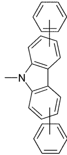
화학식 (Ar1-15)
