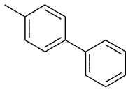
화학식 (Ar-2a)
