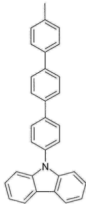
화학식 (Ar-31)
