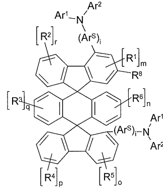
화학식 (11)
