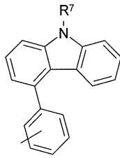
화학식 (Ar-15d)
