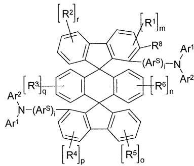
화학식 (16)
