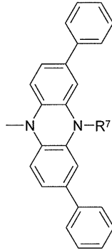
화학식 (Ar1-10a)
