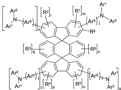
화학식 (1)
