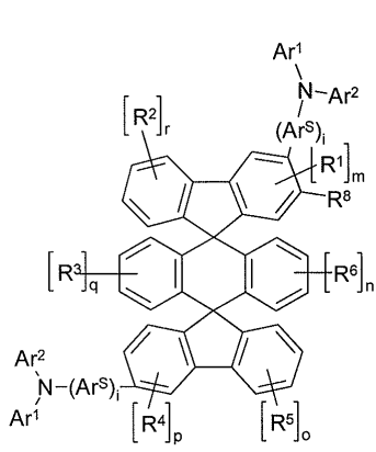
화학식 (24)
