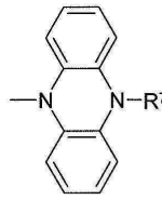
화학식 (Ar1-2)
