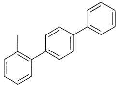
화학식 (Ar-3c)
