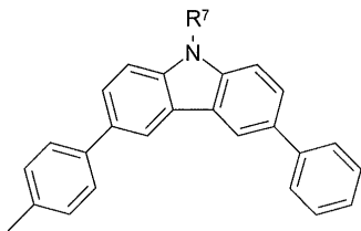
화학식 (Ar-19c)
