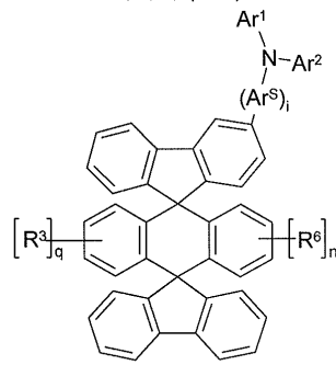
화학식 (19a)
