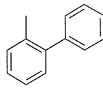
화학식 (Ar-2c)
