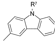
화학식 (Ar-11c)
