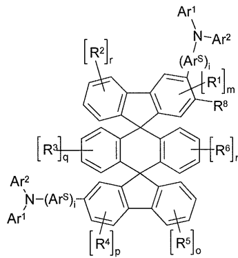
화학식 (27)
