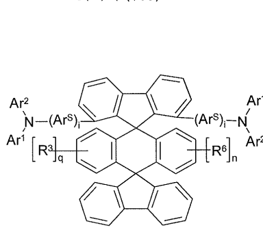
화학식 (18a)
