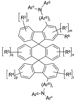
화학식 (8)
