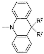
화학식 (Ar1-1)
