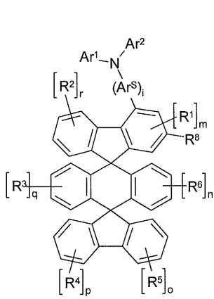
화학식 (6)
