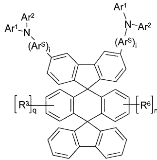
화학식 (22a)
