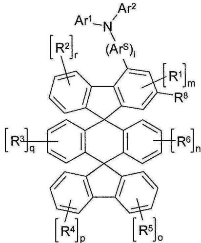
화학식 (6)
