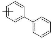
화학식 (Ar-2)
