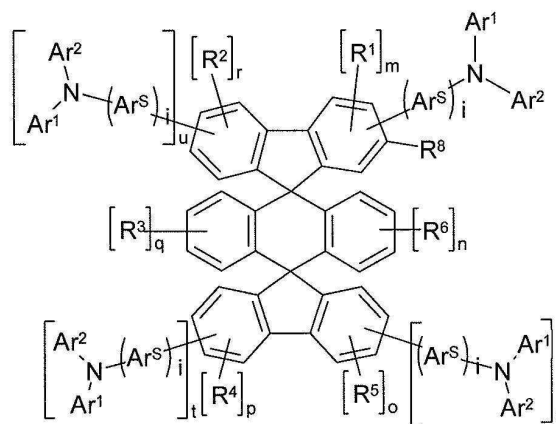
화학식 (1)
