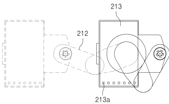
도면7
