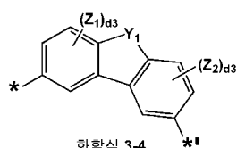
화학식 3-4
