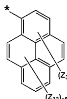
화학식 5-10
