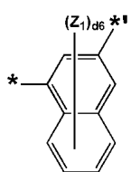
화학식 3-13
