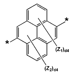
화학식 3-20
