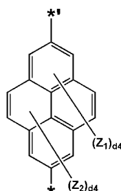
화학식 3-21
