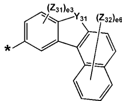
화학식 5-17
