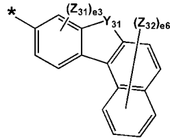
화학식 5-18
