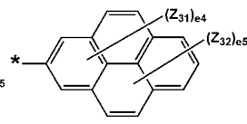
화학식 5-12
