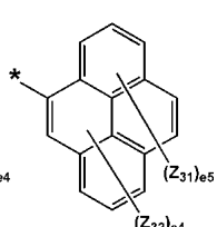
화학식 5-11
