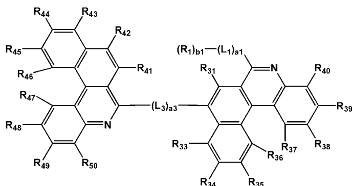
<화학식 1-8>
