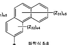
화학식 5-8
