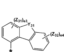
화학식 5-16
