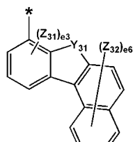
화학식 5-19
