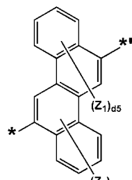
화학식 3-22
