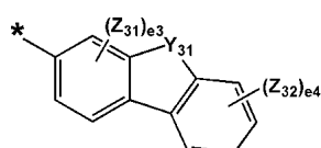
화학식 5-14
