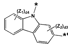
화학식 3-24
