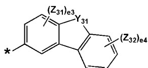
화학식 5-13
