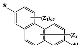
화학식 3-10
