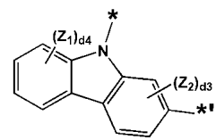
화학식 3-24
