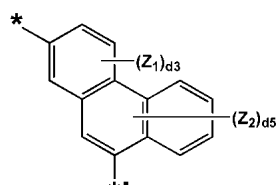
화학식 3-15
