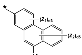
화학식 3-15
