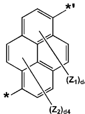
화학식 3-19
