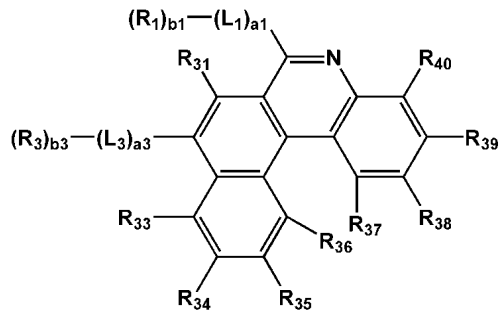
<화학식 1-4>
