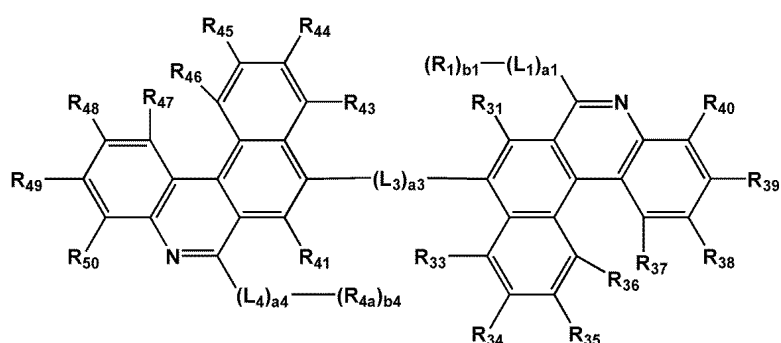
<화학식 1-8>
