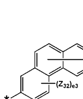
화학식 5-9
