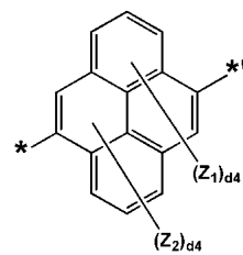
화학식 3-20
