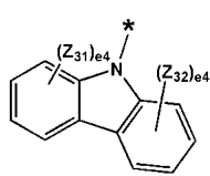
화학식 5-20
