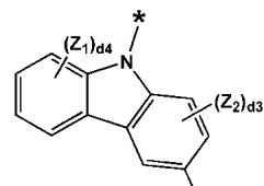
화학식 3-16
