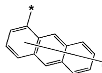
화학식 5-5
