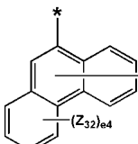
화학식 5-7
