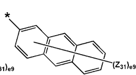
화학식 5-6
