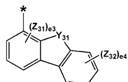
화학식 5-15
