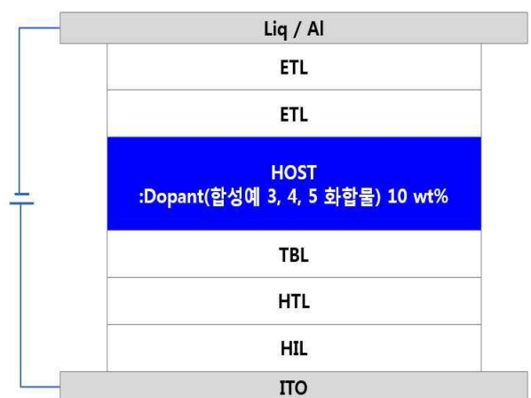
실시예 2_소자구조
