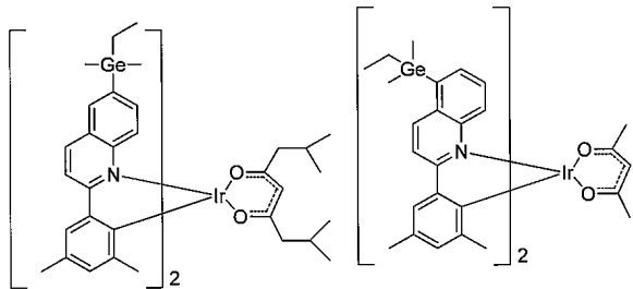
화합물 47
