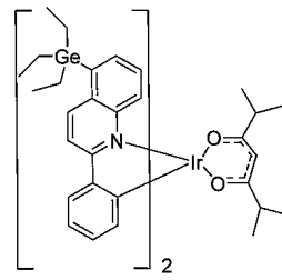
화합물 23
