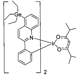
화합물 23
