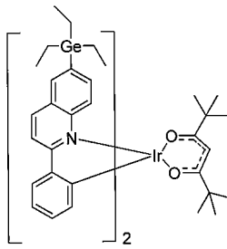
화합물 20
