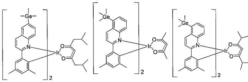
화합물 33
