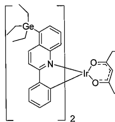
화합물 22
