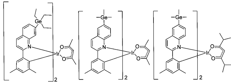
화합물 30
