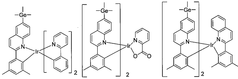
화합물 42
