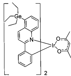
화합물 21
