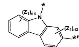
화학식 3-32
