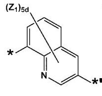
화학식 3-46
