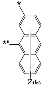
화학식 3-38
