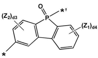
화학식 3-49
