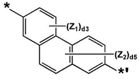
화학식 3-25
