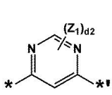
화학식 3-23
