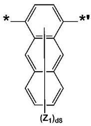
화학식 3-36
