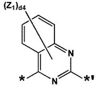
화학식 3-28
