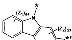
화학식 3-32
