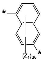
화학식 3-45
