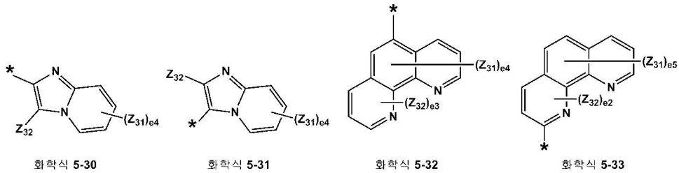
화학식 5-30
