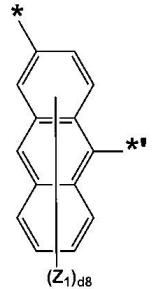
화학식 3-39
