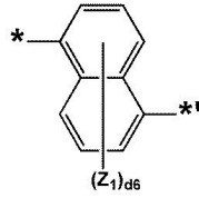
화학식 3-7
