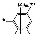
화학식 3-29
