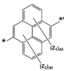
화학식 3-41
