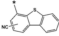
화학식 6-39
