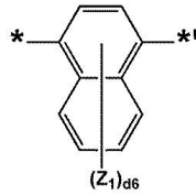
화학식 3-6
