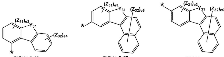
화학식 5-16
