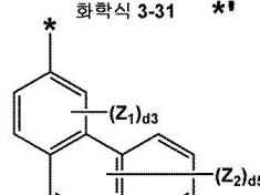
화학식 3-35
