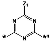
화학식 3-24
