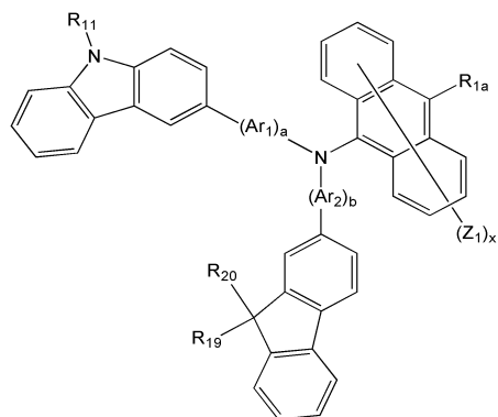
<화학식 1K>
