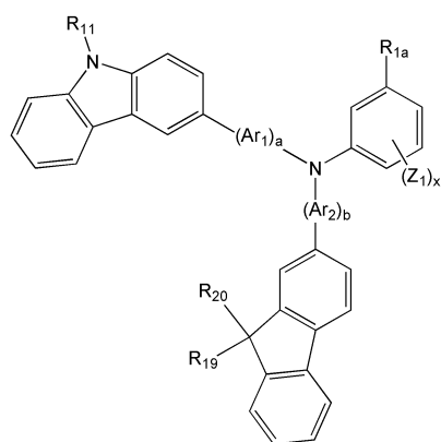
<화학식 1G>
