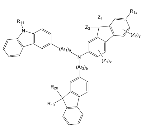
<화학식 1I>
