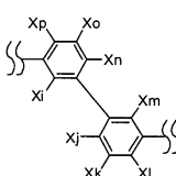
[화학식 16]
