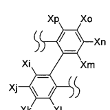
[화학식 17]
