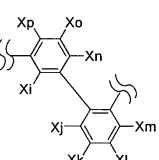
[화학식 18]
