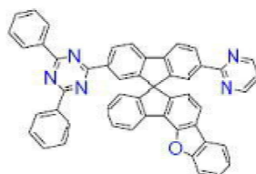
[화학식 B-116]
