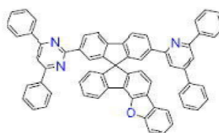
[화학식 B-125]
