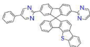
[화학식 B-191]
