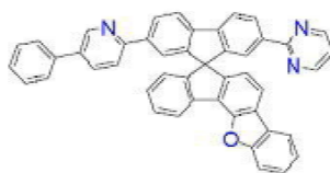
[화학식 B-63]
