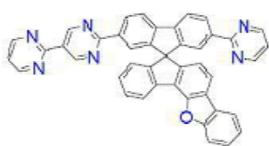
[화학식 B-82]
