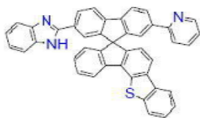
[화학식 B-180]
