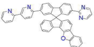
[화학식 B-74]
