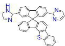
[화학식 B-178]
