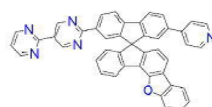
[화학식 B-81]
