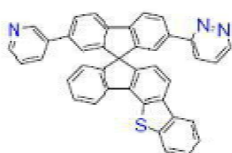
[화학식 B-150]
