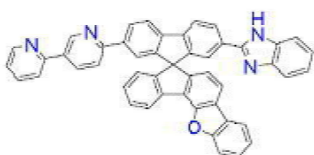
[화학식 B-76]
