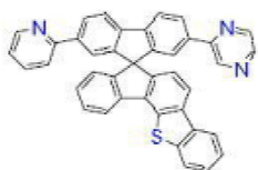
[화학식 B-149]
