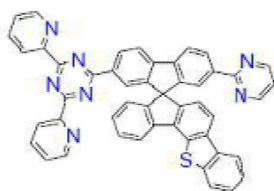
[화학식 B-245]
