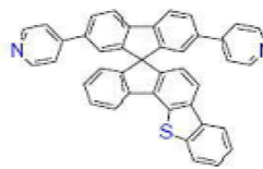
[화학식 B-143]
