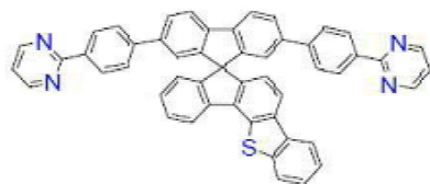
[화학식 B-220]
