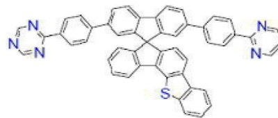
[화학식 B-223]
