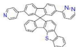
[화학식 B-156]
