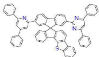
[화학식 B-249]
