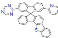
[화학식 B-170]
