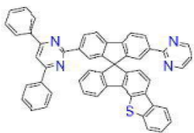
[화학식 B-236]
