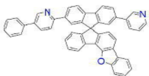
[화학식 B-61]
