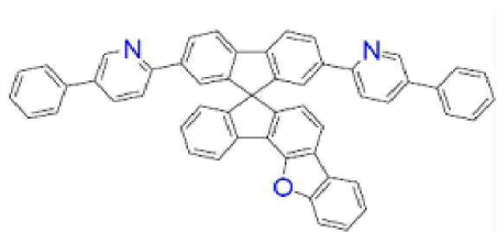
[화학식 B-86]
