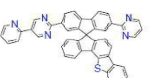
[화학식 B-204]
