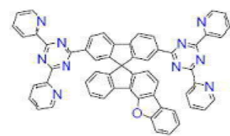
[화학식 B-132]
