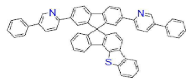
[화학식 B-211]
