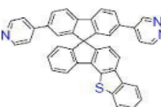
[화학식 B-157]
