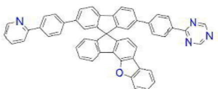
[화학식 B-92]
