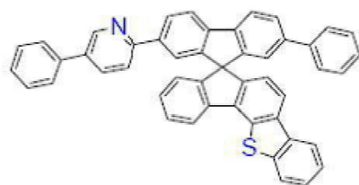
[화학식 B-184]
