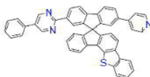
[화학식 B-190]
