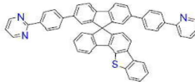
[화학식 B-219]
