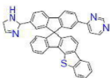
[화학식 B-177]
