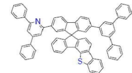
[화학식 B-246]
