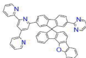
[화학식 B-107]
