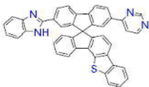
[화학식 B-182]
