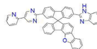
[화학식 B-80]
