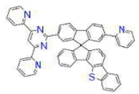
[화학식 B-238]
