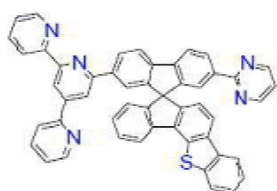
[화학식 B-233]
