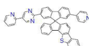
[화학식 B-203]
