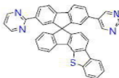
[화학식 B-165]
