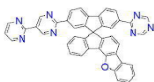
[화학식 B-83]
