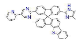
[화학식 B-206]
