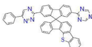
[화학식 B-198]
