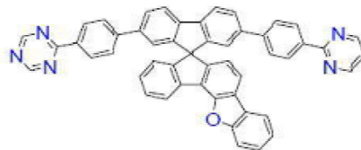
[화학식 B-97]
