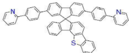
[화학식 B-216]
