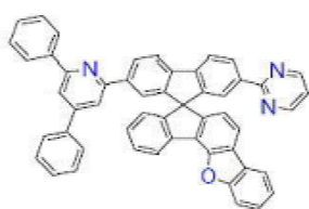
[화학식 B-103]
