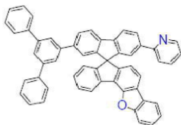
[화학식 B-100]
