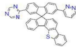
[화학식 B-168]
