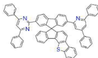
[화학식 B-251]
