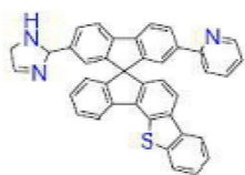
[화학식 B-176]
