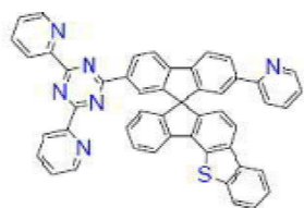
[화학식 B-244]
