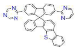
[화학식 B-172]
