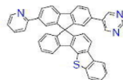
[화학식 B-147]
