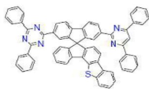
[화학식 B-255]
