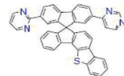
[화학식 B-164]
