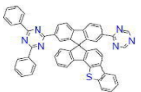
[화학식 B-243]
