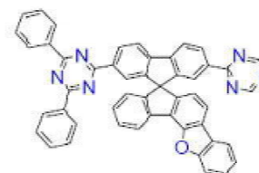
[화학식 B-117]
