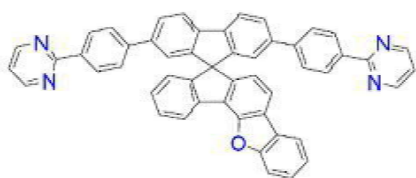
[화학식 B-94]
