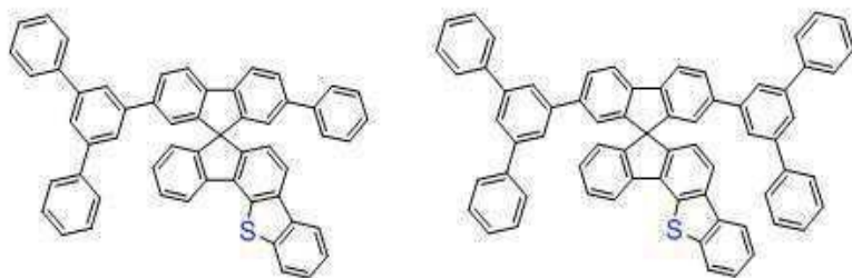
[화학식 A-21]
