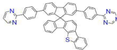
[화학식 B-221]
