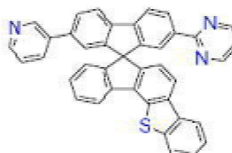
[화학식 B-154]
