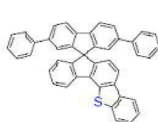
[화학식 A-17]
