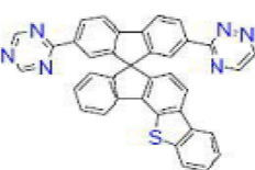
[화학식 B-174]
