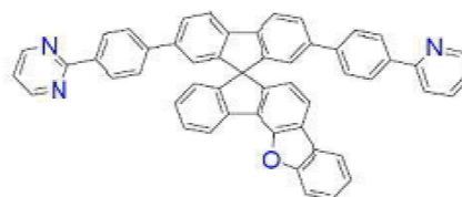
[화학식 B-93]
