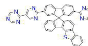
[화학식 B-209]
