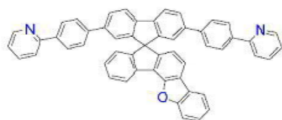
[화학식 B-90]
