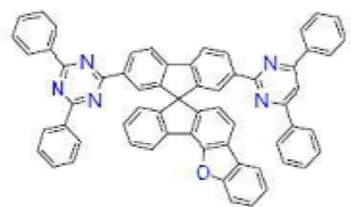
[화학식 B-129]
