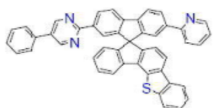
[화학식 B-192]
