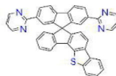
[화학식 B-166]
