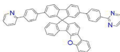
[화학식 B-91]
