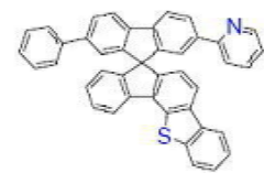
[화학식 B-136]
