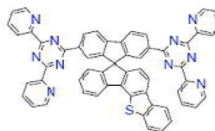
[화학식 B-255]
