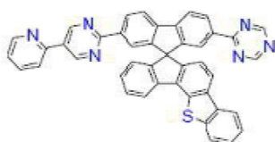
[화학식 B-205]
