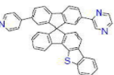
[화학식 B-161]
