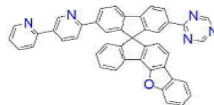
[화학식 B-75]
