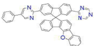
[화학식 B-69]
