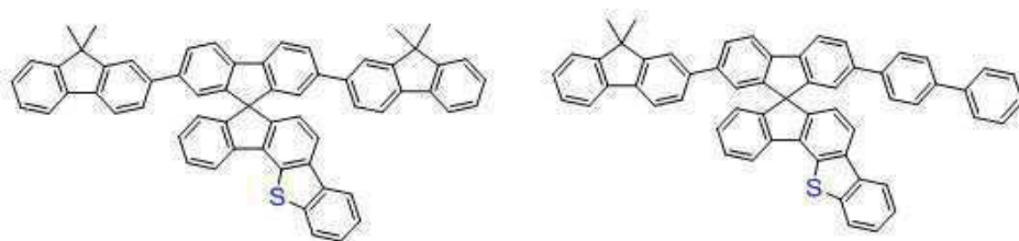
[화학식 A-23]
