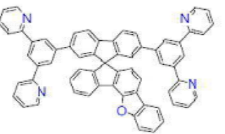
[화학식 B-131]
