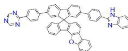
[화학식 B-97]
