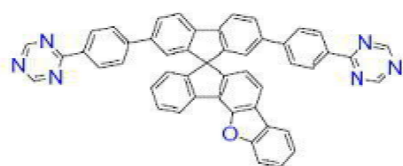
[화학식 B-98]
