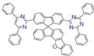
[화학식 B-127]
