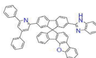
[화학식 B-105]
