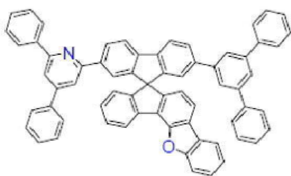
[화학식 B-120]
