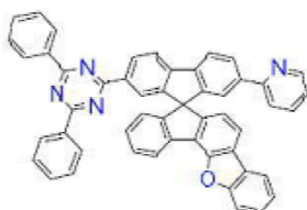
[화학식 B-115]
