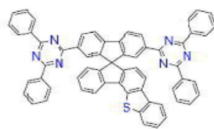
[화학식 B-256]
