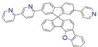
[화학식 B-73]
