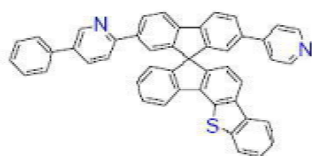
[화학식 B-188]
