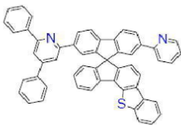
[화학식 B-228]
