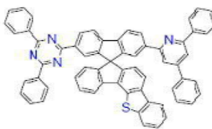
[화학식 B-251]
