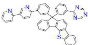
[화학식 B-201]
