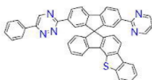
[화학식 B-197]
