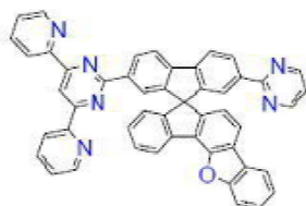
[화학식 B-113]
