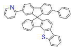
[화학식 B-137]
