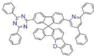
[화학식 B-128]
