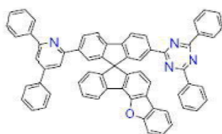
[화학식 B-124]
