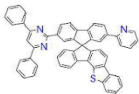
[화학식 B-235]
