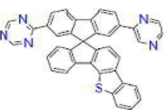
[화학식 B-173]
