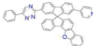
[화학식 B-70]
