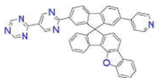
[화학식 B-85]
