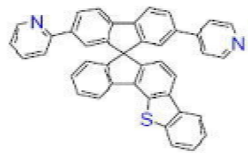
[화학식 B-140]
