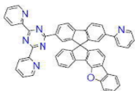
[화학식 B-118]
