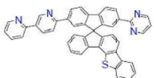
[화학식 B-200]
