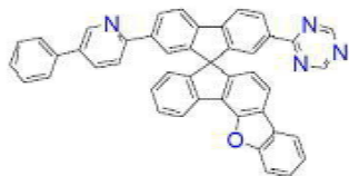
[화학식 B-64]
