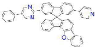
[화학식 B-67]
