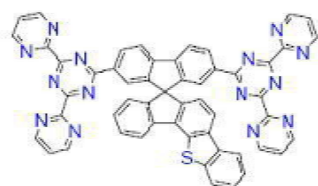
[화학식 B-256]
