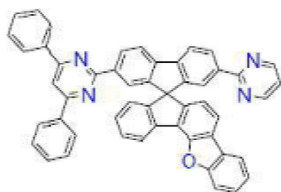
[화학식 B110]
