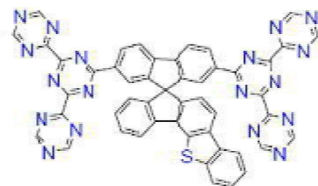
[화학식 B-257]
