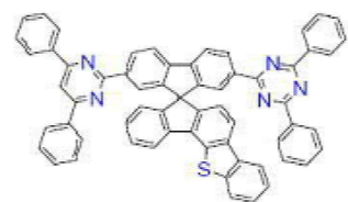
[화학식 B-253]
