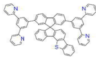
[화학식 B-257]
