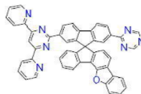
[화학식 B-114]
