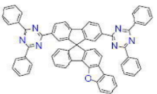
[화학식 B-130]
