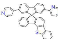
[화학식 B-158]
