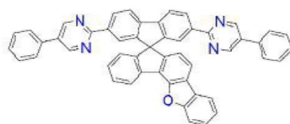
[화학식 B-89]
