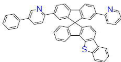
[화학식 B-186]
