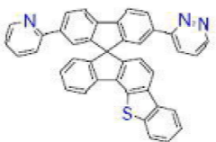
[화학식 B-144]
