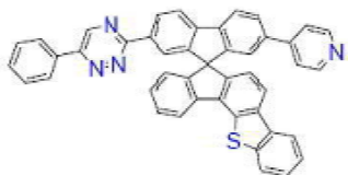
[화학식 B-196]
