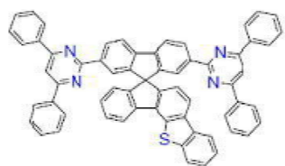
[화학식 B-252]
