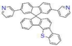
[화학식 B-141]
