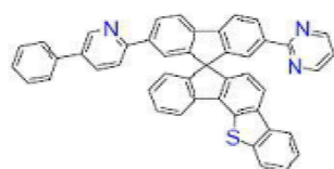
[화학식 B-186]
