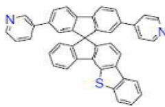
[화학식 B-142]
