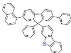
[화학식 A-18]
