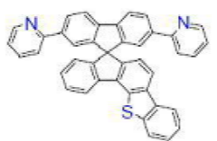
[화학식 B-138]
