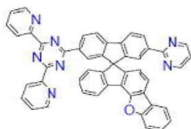
[화학식 B-119]
