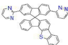
[화학식 B-162]
