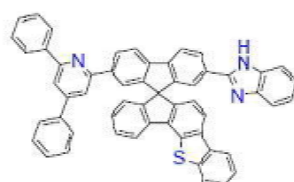
[화학식 B-231]
