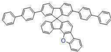
[화학식 A-8]
