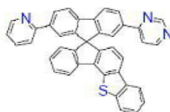
[화학식 B-146]
