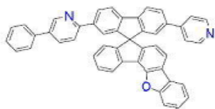
[화학식 B-62]
