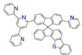
[화학식 B-232]
