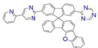
[화학식 B-79]
