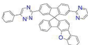
[화학식 B-71]
