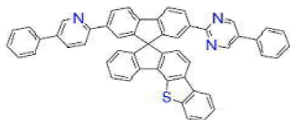
[화학식 B-214]
