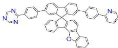
[화학식 B-96]
