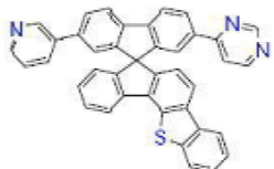
[화학식 B-152]
