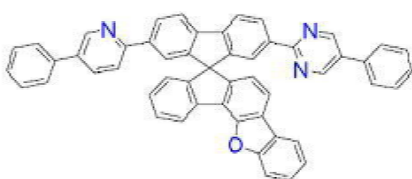
[화학식 B-88]
