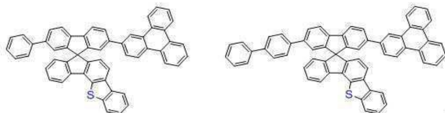
[화학식 A-23]
