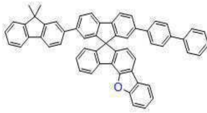
[화학식 A-10]
