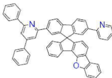
[화학식 B-102]
