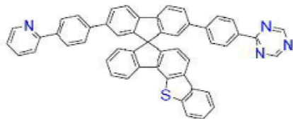
[화학식 B-218]
