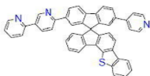
[화학식 B-199]
