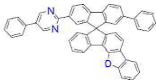
[화학식 B-65]
