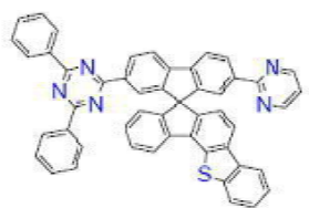
[화학식 B-242]
