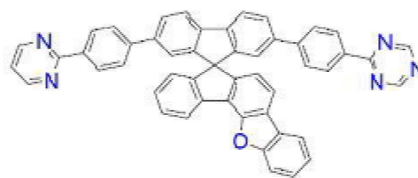
[화학식 B-95]
