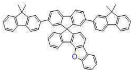
[화학식 A-11]
