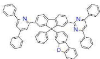
[화학식 B-123]
