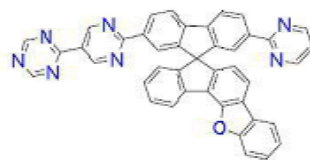
[화학식 B-83]
