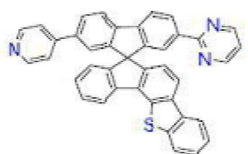
[화학식 B-160]
