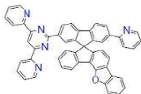
[화학식 B-112]
