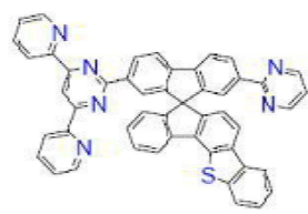
[화학식 B-239]
