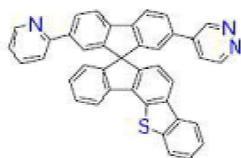
[화학식 B-145]
