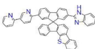
[화학식 B-202]
