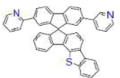
[화학식 B-139]
