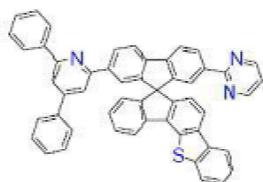
[화학식 B-229]
