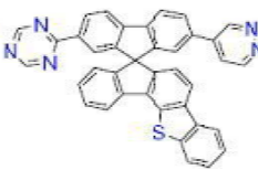
[화학식 B-169]
