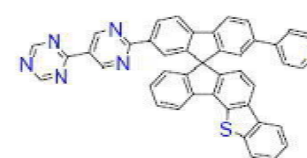
[화학식 B-211]
