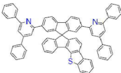
[화학식 B-248]
