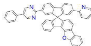
[화학식 B-66]
