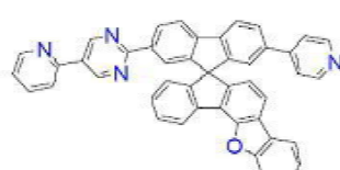
[화학식 B-77]
