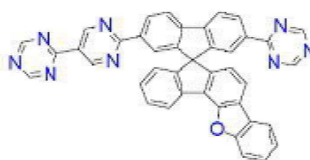
[화학식 B-84]
