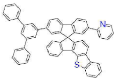
[화학식 B-226]
