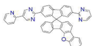
[화학식 B-78]
