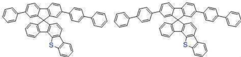
[화학식 A-19]
