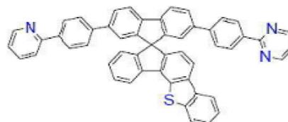
[화학식 B-217]
