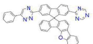
[화학식 B-72]
