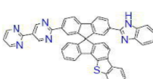
[화학식 B-207]
