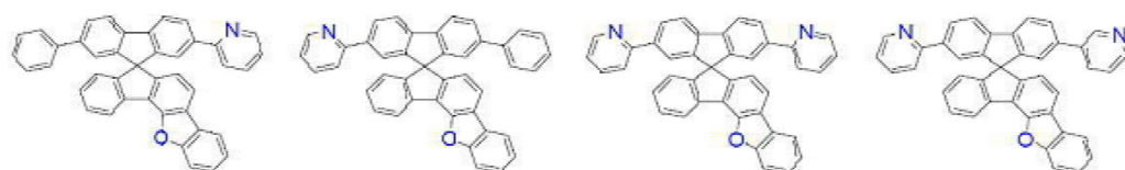
[화학식 B-5]
