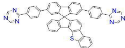
[화학식 B-224]
