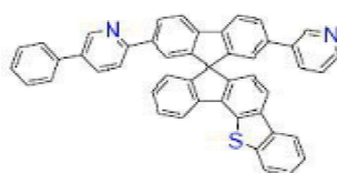
[화학식 B-187]
