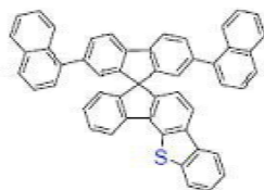
[화학식 A-15]
