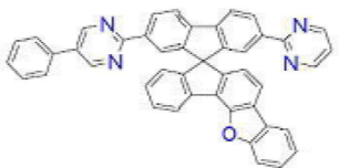
[화학식 B-68]
