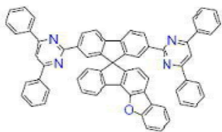
[화학식 B-126]
