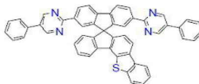
[화학식 B-215]
