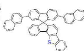
[화학식 A-16]
