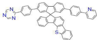
[화학식 B-222]
