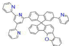
[화학식 B-106]
