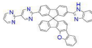
[화학식 B-84]
