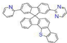
[화학식 B-148]
