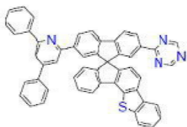
[화학식 B-230]
