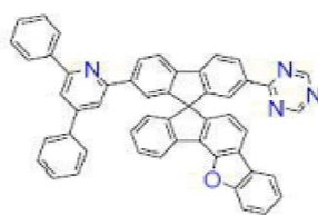
[화학식 B-104]
