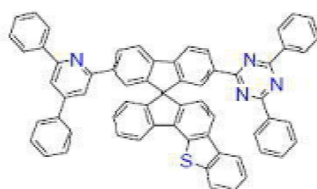
[화학식 B-250]
