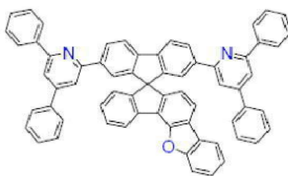
[화학식 B-122]
