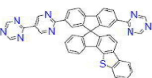
[화학식 B-210]
