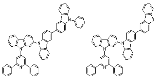
[화학식 B-16] [화학식 B-18]
