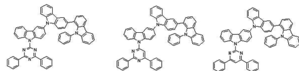
[화학식 A-25] [화학식 A-26] [화학식 A-27]
