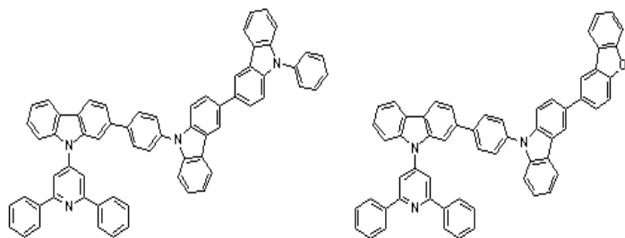
[화학식 B-31] [화학식 B-33]
