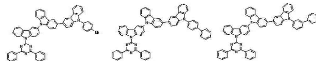
[화학식 A-67] [화학식 A-68] [화학식 A-69]
