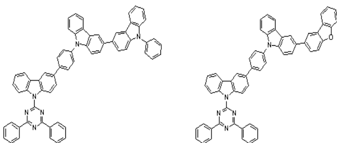
[화학식 A-37] [화학식 A-39]
