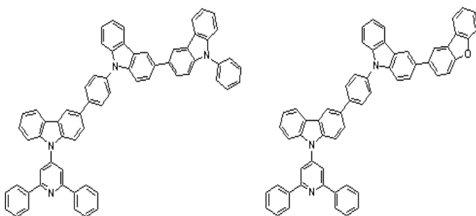
[화학식 A-49] [화학식 A-51]
