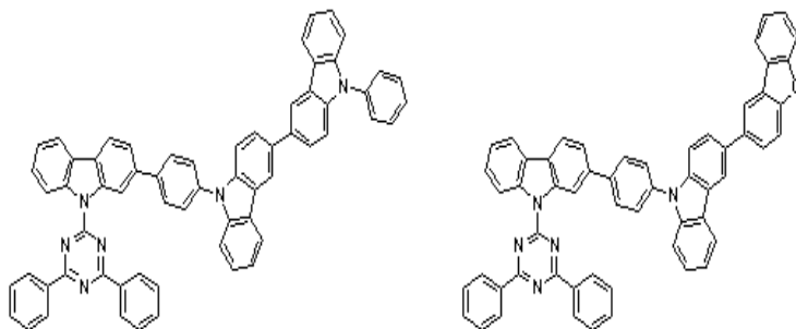
[화학식 B-19] [화학식 B-21]
