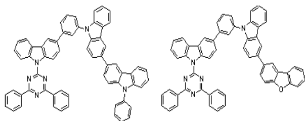
[화학식 A-52] [화학식 A-54]
