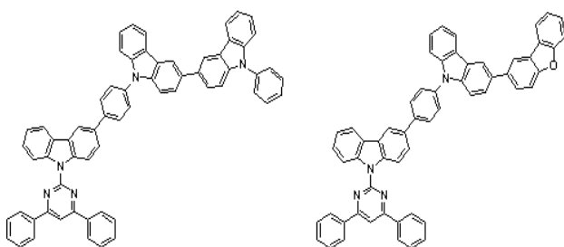
[화학식 A-40] [화학식 A-42]
