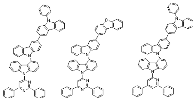
[화학식 B-49] [화학식 B-50] [화학식 B-51]
