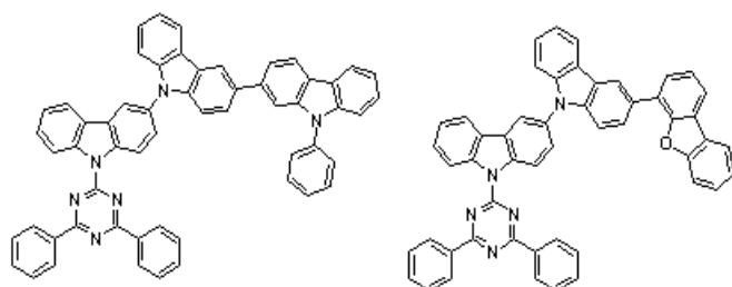
[화학식 A-16] [화학식 A-18]
