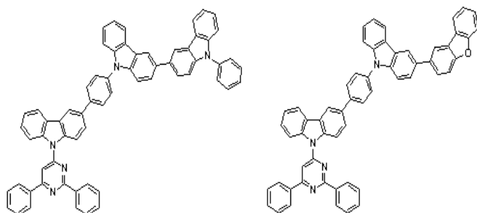
[화학식 A-40] [화학식 A-42]
