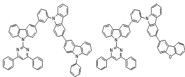
[화학식 A-55] [화학식 A-57]
