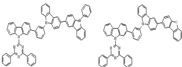
[화학식 B-34] [화학식 B-36]
