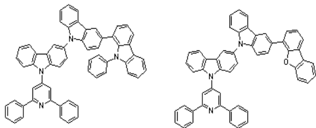
[화학식 A-31] [화학식 A-33]
