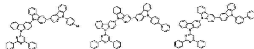
[화학식 A-70] [화학식 A-71] [화학식 A-72]
