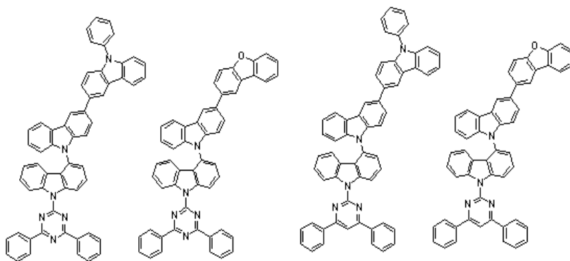
[화학식 B-49] [화학식 B-50] [화학식 B-51]
