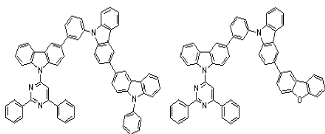
[화학식 A-55] [화학식 A-57]
