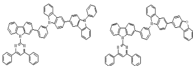
[화학식 B-37] [화학식 B-39]
