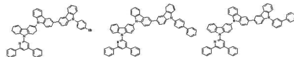
[화학식 A-73] [화학식 A-74] [화학식 A-75]
