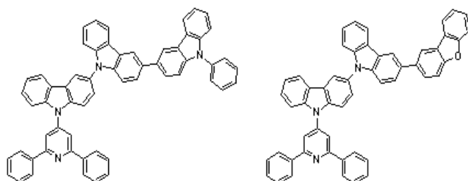
[화학식 A-34] [화학식 A-36]
