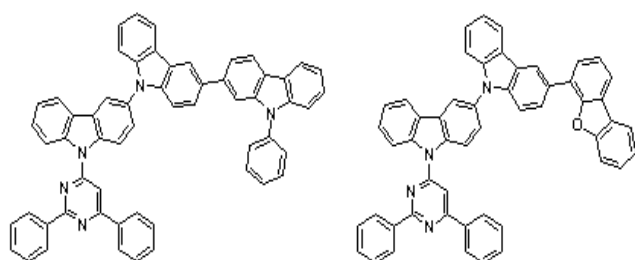
[화학식 A-22] [화학식 A-24]
