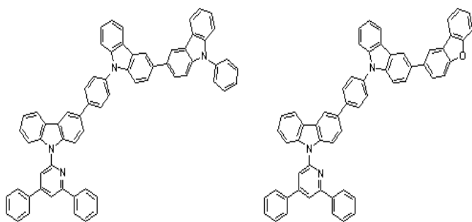
[화학식 A-46] [화학식 A-48]
