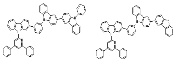
[화학식 B-43] [화학식 B-45]
