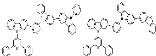
[화학식 B-46] [화학식 B-47] [화학식 B-48][화학식 B-85]
