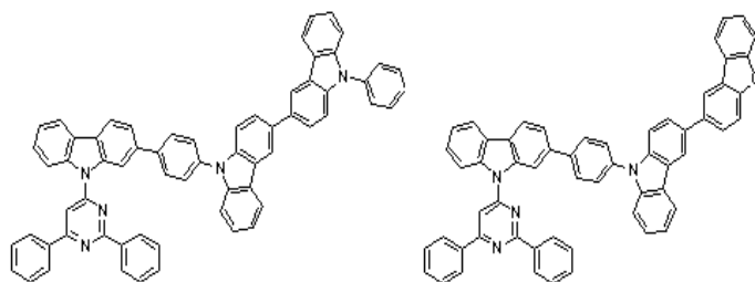
[화학식 B-22] [화학식 B-24]
