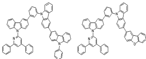
[화학식 A-61] [화학식 A-63]
