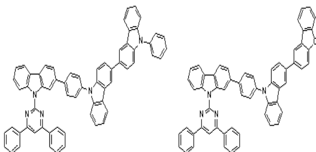
[화학식 B-22] [화학식 B-24]
