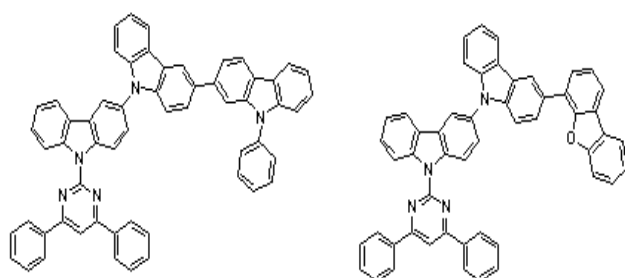
[화학식 A-16] [화학식 A-18]
