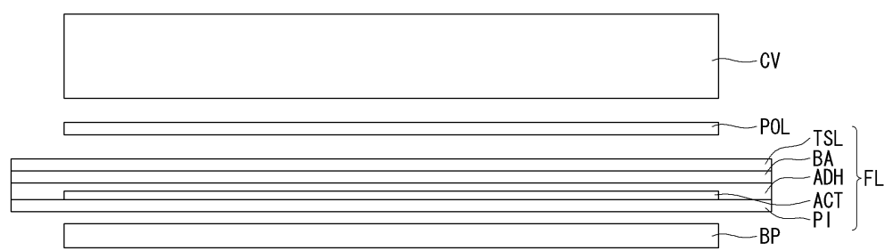
도면5
