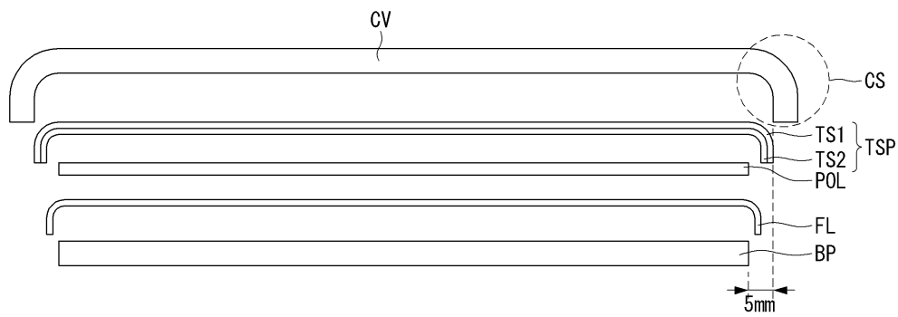
도면3
