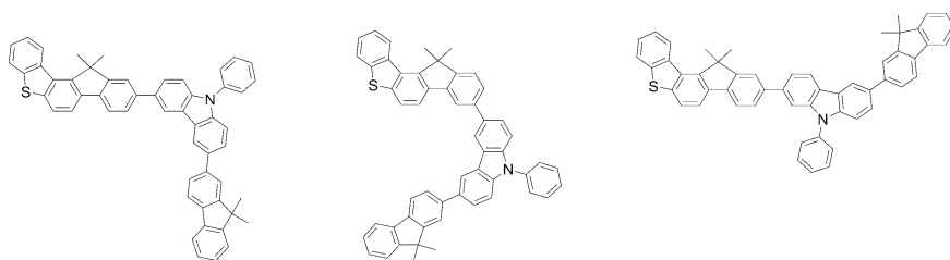
[화학식 D-97] [화학식 D-98] [화학식 D-99]
