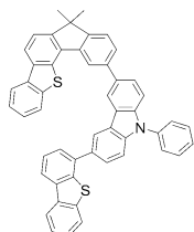
[화학식 D-78]
