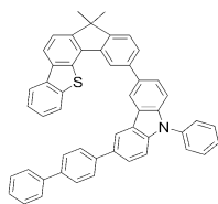
[화학식 D-34] [화학식 D-35] [화학식 D-36]
