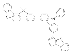
[화학식 D-76] [화학식 D-77]
