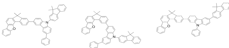
[화학식 D-100] [화학식 D-101] [화학식 D-102]
