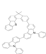
[화학식 D-142] [화학식 D-143] [화학식 D-144]
