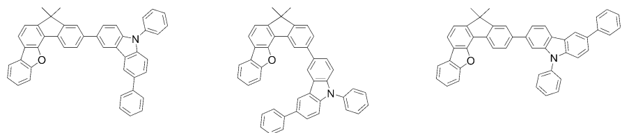
[화학식 D-16] [화학식 D-17] [화학식 D-18]
