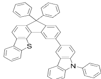
[화학식 D-133] [화학식 D-134] [화학식 D-135]
