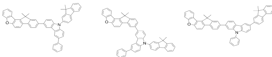
[화학식 D-103] [화학식 D-104] [화학식 D-105]
