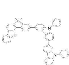
[화학식 D-142] [화학식 D-143] [화학식 D-144]
