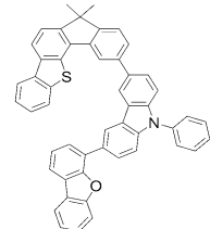
[화학식 D-84]
