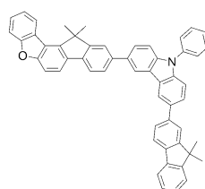
[화학식 D-88] [화학식 D-89]
