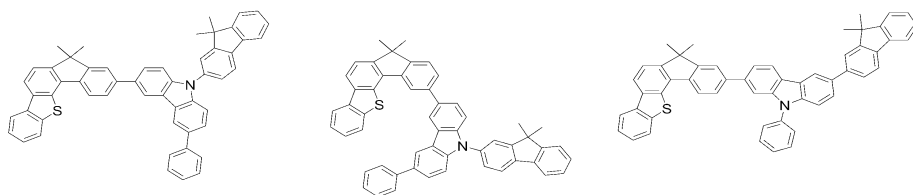
[화학식 D-106] [화학식 D-107] [화학식 D-108]
