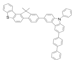
[화학식 D-37] [화학식 D-38] [화학식 D-39]
