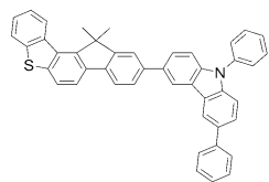
[화학식 D-22] [화학식 D-23] [화학식 D-24]
