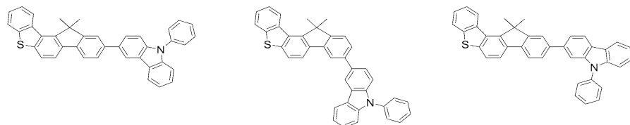
[화학식 D-13] [화학식 D-14] [화학식 D-15]
