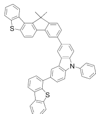
[화학식 D-81]
