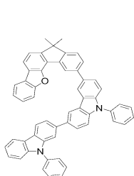
[화학식 D-142] [화학식 D-143] [화학식 D-144]
