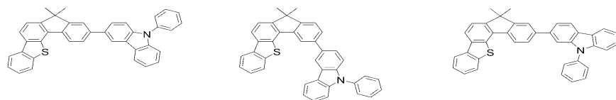
[화학식 D-10] [화학식 D-11] [화학식 D-12]
