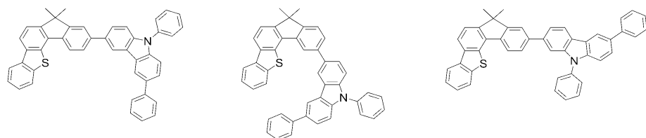
[화학식 D-19] [화학식 D-20] [화학식 D-21]
