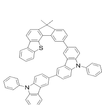
[화학식 D-139] [화학식 D-140] [화학식 D-141]
