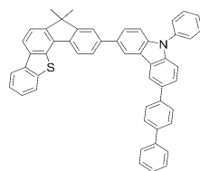
[화학식 D-34] [화학식 D-35] [화학식 D-36]
