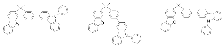
[화학식 D-4] [화학식 D-5] [화학식 D-6]
