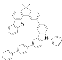
[화학식 D-28] [화학식 D-29] [화학식 D-30]
