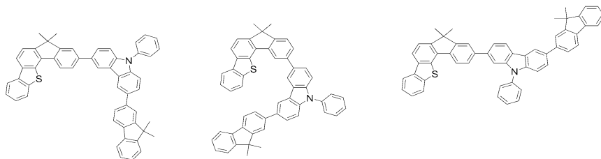
[화학식 D-94] [화학식 D-95] [화학식 D-96]
