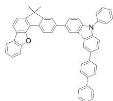
[화학식 D-31] [화학식 D-32] [화학식 D-33]
