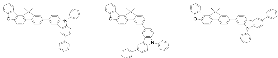
[화학식 D-19] [화학식 D-20] [화학식 D-21]
