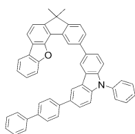
[화학식 D-31] [화학식 D-32] [화학식 D-33]
