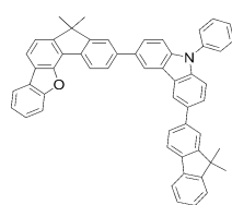
[화학식 D-88] [화학식 D-89]
