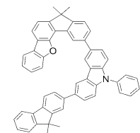
[화학식 D-90]
