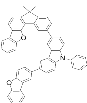
[화학식 D-37] [화학식 D-38] [화학식 D-39]
