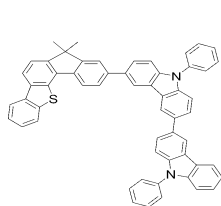
[화학식 D-139] [화학식 D-140] [화학식 D-141]
