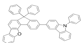
[화학식 D-127] [화학식 D-128] [화학식 D-129]
