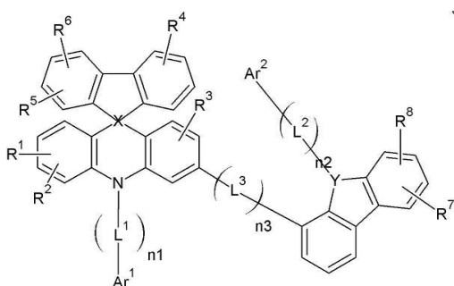
[화학식 4-3]
