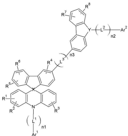
[화학식 2-4]
