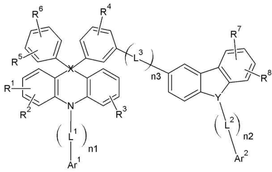
[화학식 1-2]
