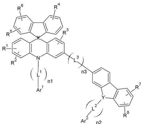
[화학식 4-3]
