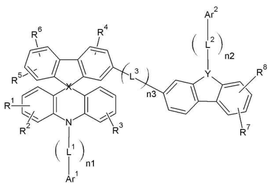
[화학식 2-3]
