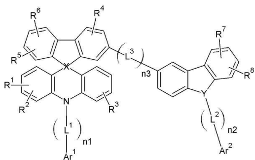
[화학식 2-2]
