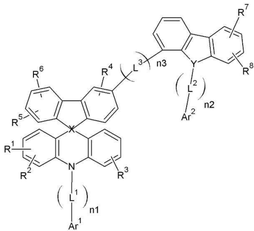
[화학식 3-1]
