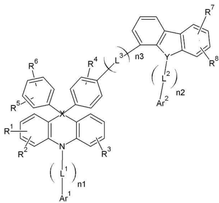
[화학식 1-6]
