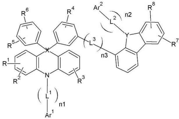
[화학식 1-3]
