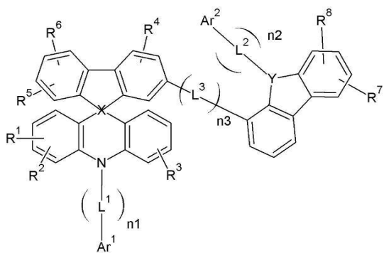
[화학식 2-4]
