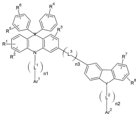
[화학식 3-1]
