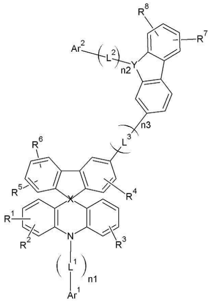
[화학식 2-6]
