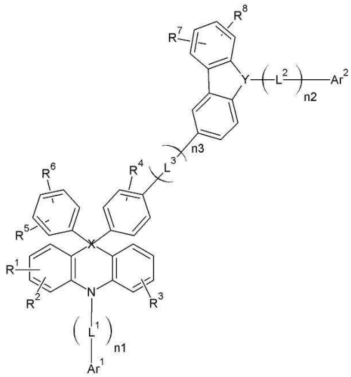
[화학식 1-5]
