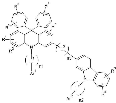
[화학식 3-3]
