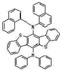
[화학식 A-97] [화학식 A-98] [화학식 A-99] [화학식 A-100]
