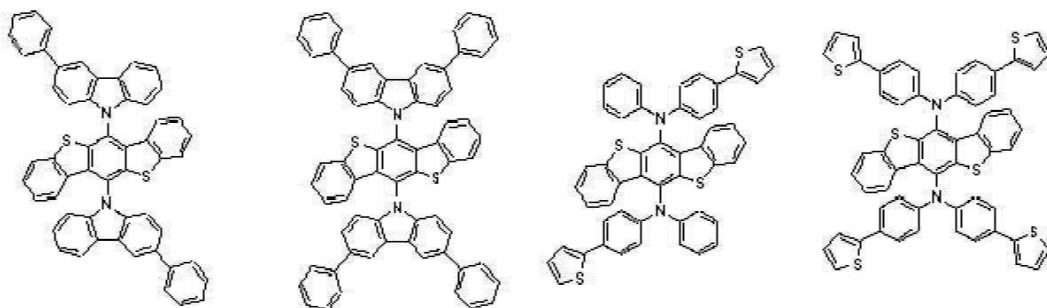
[화학식 A-69] [화학식 A-70] [화학식 A-71] [화학식 A-72]
