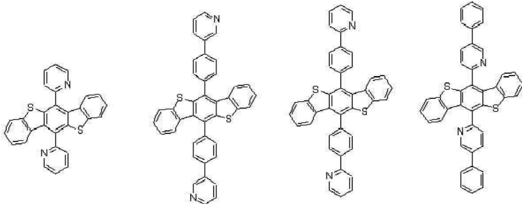
[화학식 B-17] [화학식 B-18] [화학식 B-19] [화학식 B-20]
