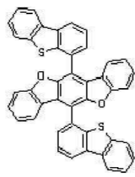
[화학식 A-113] [화학식 A-114] [화학식 A-115] [화학식 A-116]
