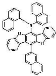
[화학식 A-45] [화학식 A-46] [화학식 A-47] [화학식 A-48]
