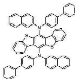
[화학식 A-61] [화학식 A-62] [화학식 A-63] [화학식 A-64]
