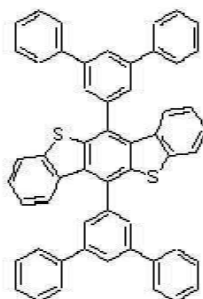
[화학식 A-121] [화학식 A-122] [화학식 A-123] [화학식 A-124]
