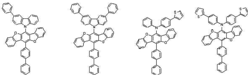
[화학식 A-41] [화학식 A-42] [화학식 A-43] [화학식 A-44]
