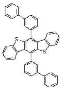
[화학식 A-125] [화학식 A-126] [화학식 A-127] [화학식 A-128]
