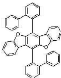
[화학식 A-105] [화학식 A-106] [화학식 A-107] [화학식 A-108]
