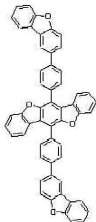
[화학식 A-117] [화학식 A-118] [화학식 A-119] [화학식 A-120]
