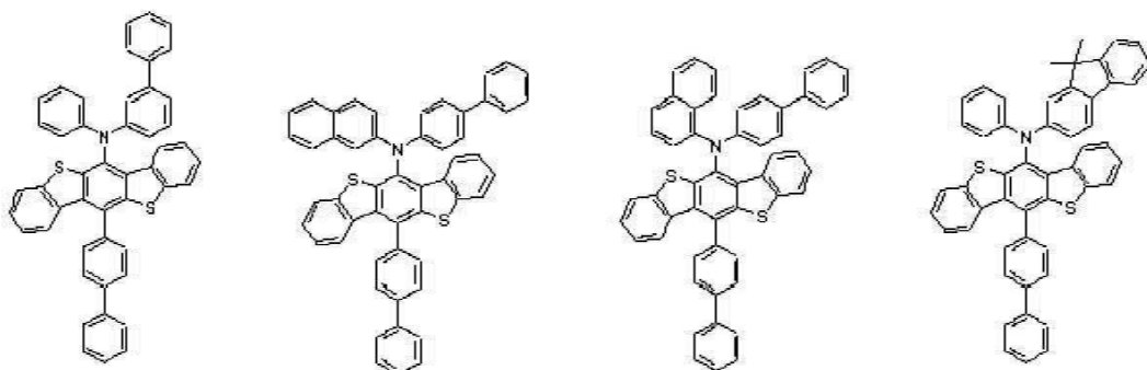
[화학식 A-77] [화학식 A-78] [화학식 A-79] [화학식 A-80]
