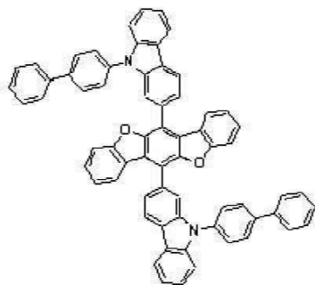
[화학식 A-105] [화학식 A-106] [화학식 A-107] [화학식 A-108]
