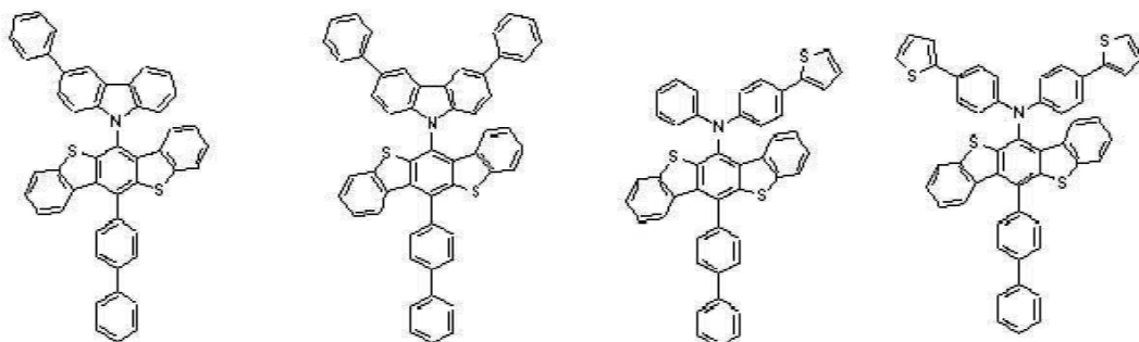
[화학식 A-89] [화학식 A-90] [화학식 A-91] [화학식 A-92]
