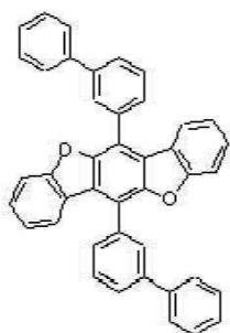
[화학식 A-105] [화학식 A-106] [화학식 A-107] [화학식 A-108]
