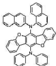
[화학식 A-49] [화학식 A-50] [화학식 A-51] [화학식 A-52]
