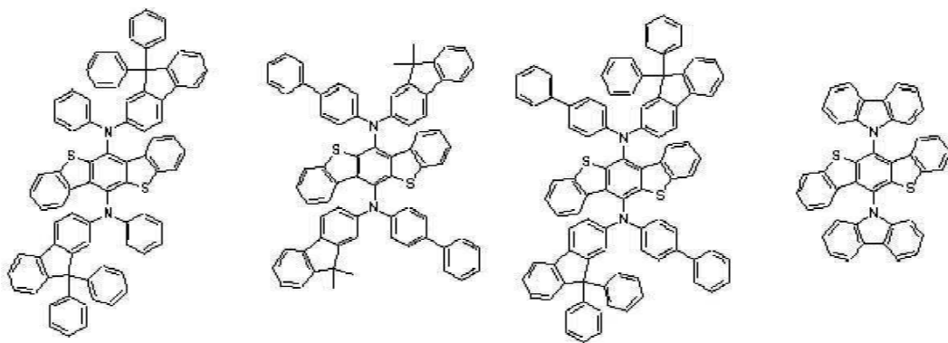
[화학식 A-65] [화학식 A-66] [화학식 A-67] [화학식 A-68]
