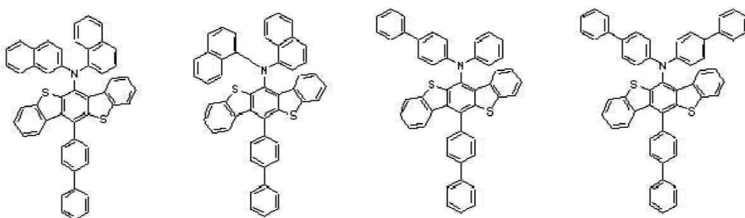
[화학식 A-73] [화학식 A-74] [화학식 A-75] [화학식 A-76]
