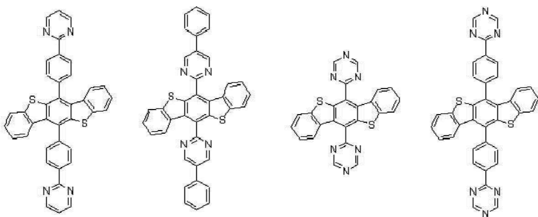
[화학식 B-21] [화학식 B-22] [화학식 B-23] [화학식 B-24]
