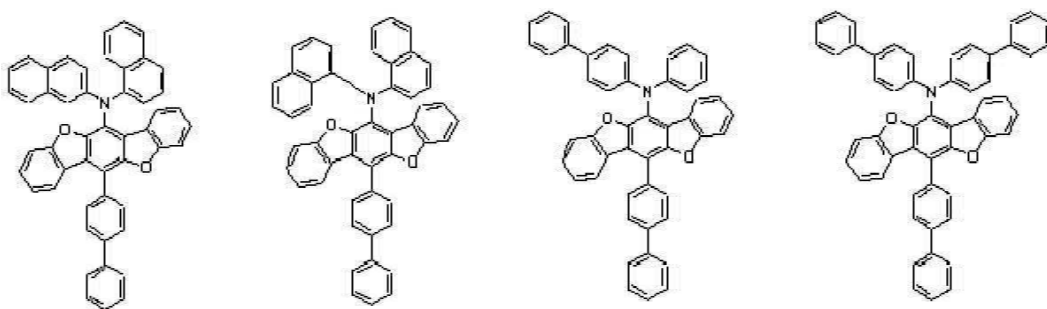
[화학식 A-25] [화학식 A-26] [화학식 A-27] [화학식 A-28]
