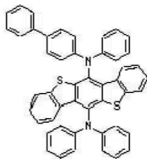
[화학식 A-97] [화학식 A-98] [화학식 A-99] [화학식 A-100]
