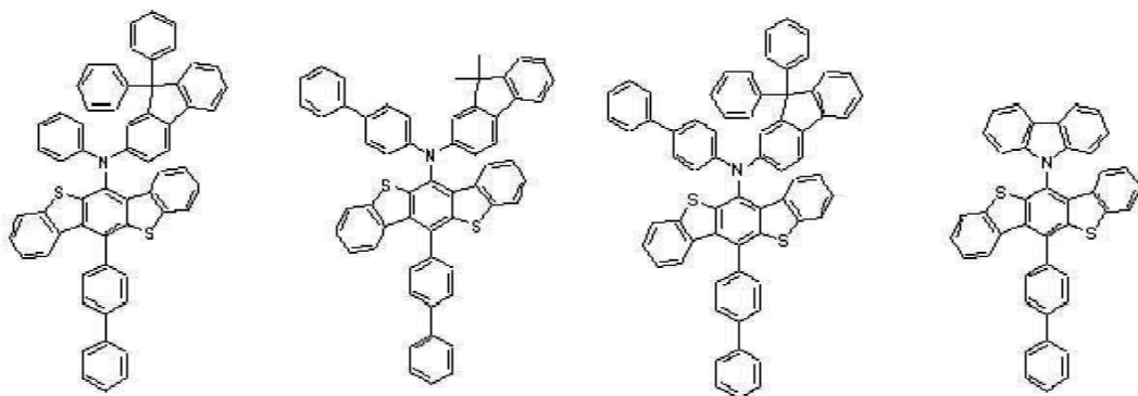
[화학식 A-85] [화학식 A-86] [화학식 A-87] [화학식 A-88]
