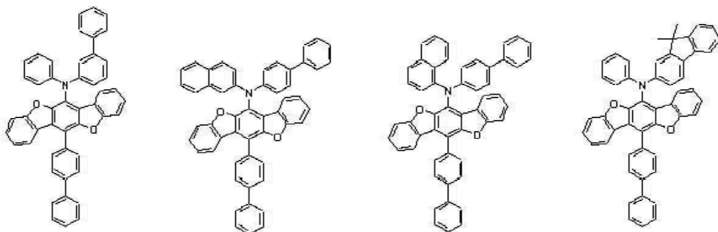
[화학식 A-29] [화학식 A-30] [화학식 A-31] [화학식 A-32]
