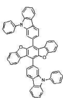
[화학식 A-109] [화학식 A-110] [화학식 A-111] [화학식 A-112]
