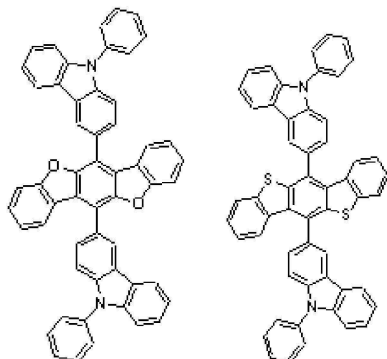
[화학식 A-137] [화학식 A-138]
