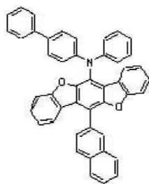
[화학식 A-45] [화학식 A-46] [화학식 A-47] [화학식 A-48]
