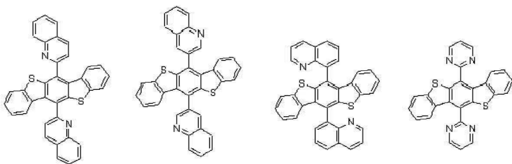
[화학식 B-21] [화학식 B-22] [화학식 B-23] [화학식 B-24]
