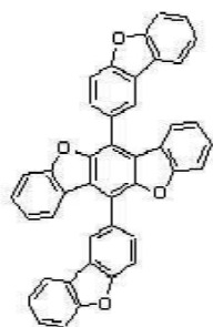
[화학식 A-113] [화학식 A-114] [화학식 A-115] [화학식 A-116]
