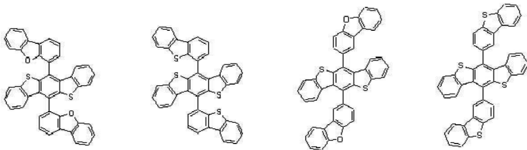
[화학식 A-133] [화학식 A-134] [화학식 A-135] [화학식 A-136]
