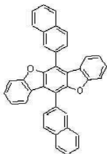
[화학식 A-101] [화학식 A-102] [화학식 A-103] [화학식 A-104]
