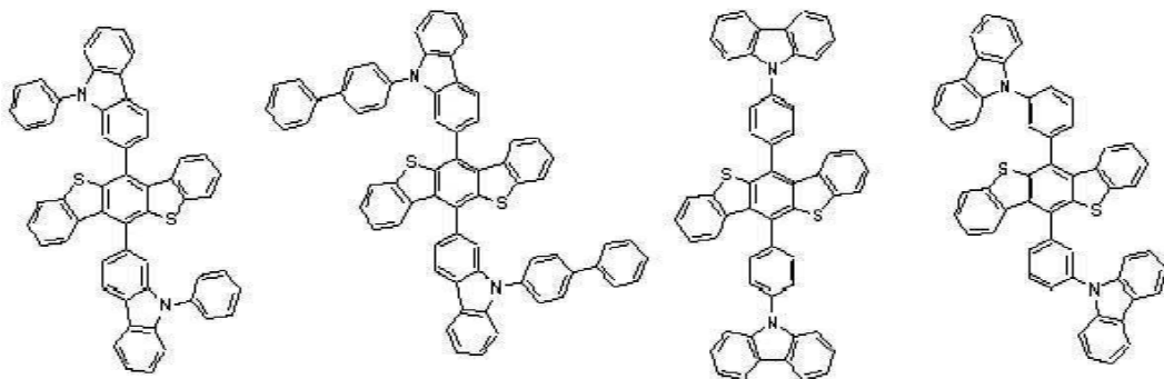
[화학식 A-129] [화학식 A-130] [화학식 A-131] [화학식 A-132]
