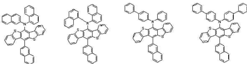
[화학식 A-93] [화학식 A-94] [화학식 A-95] [화학식 A-96]
