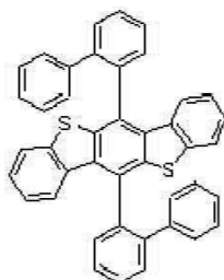
[화학식 A-125] [화학식 A-126] [화학식 A-127] [화학식 A-128]
