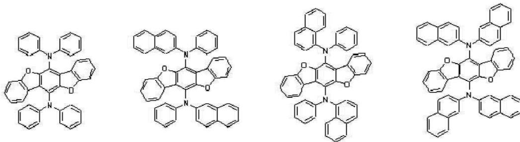
[화학식 A-13] [화학식 A-14] [화학식 A-15] [화학식 A-16]
