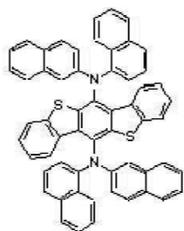
[화학식 A-57] [화학식 A-58] [화학식 A-59] [화학식 A-60]
