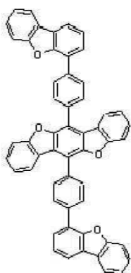
[화학식 A-117] [화학식 A-118] [화학식 A-119] [화학식 A-120]
