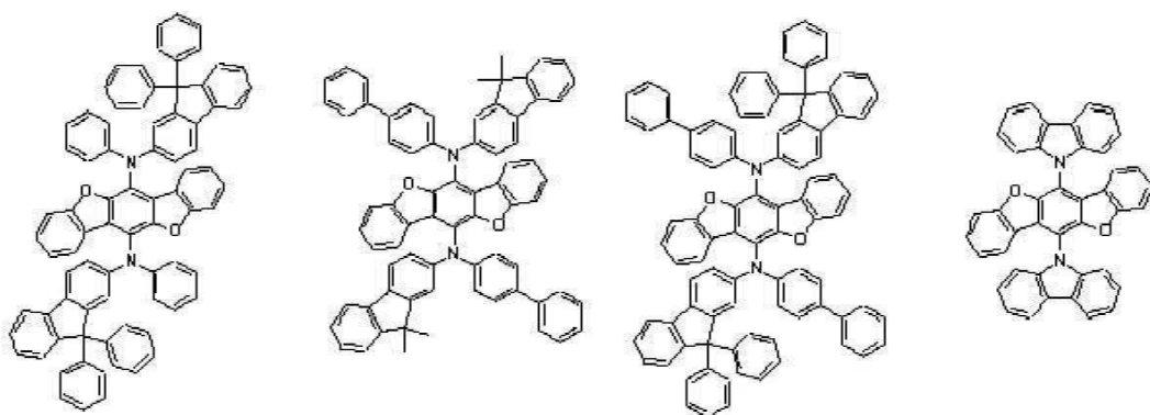
[화학식 A-17] [화학식 A-18] [화학식 A-19] [화학식 A-20]
