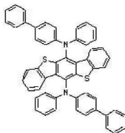
[화학식 A-57] [화학식 A-58] [화학식 A-59] [화학식 A-60]
