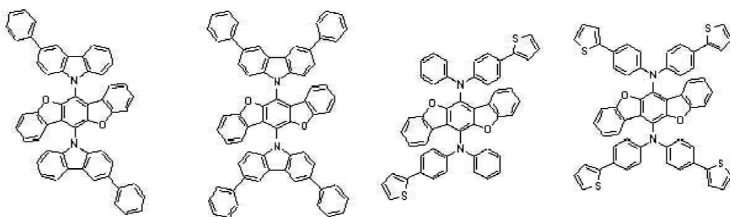
[화학식 A-21] [화학식 A-22] [화학식 A-23] [화학식 A-24]
