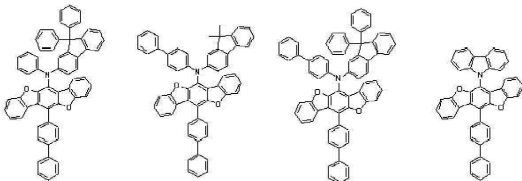
[화학식 A-37] [화학식 A-38] [화학식 A-39] [화학식 A-40]
