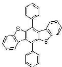
[화학식 A-121] [화학식 A-122] [화학식 A-123] [화학식 A-124]
