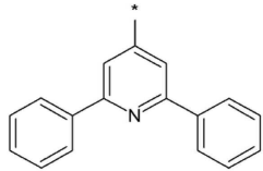
[화학식 8]
