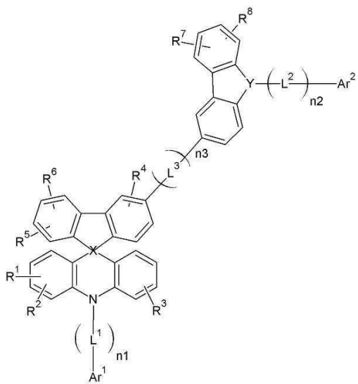
[화학식 2-4]
