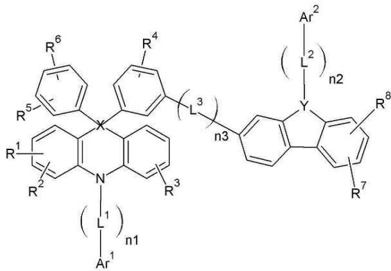
[화학식 1-3]
