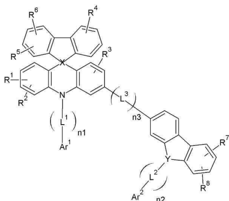
[화학식 4-3]
