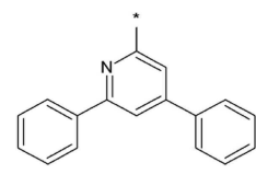
[화학식 9]
