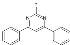
[화학식 8]
