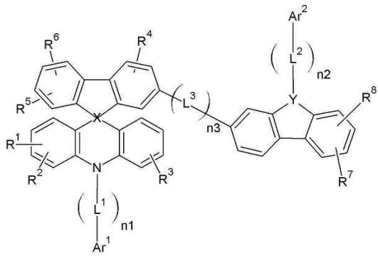
[화학식 2-3]
