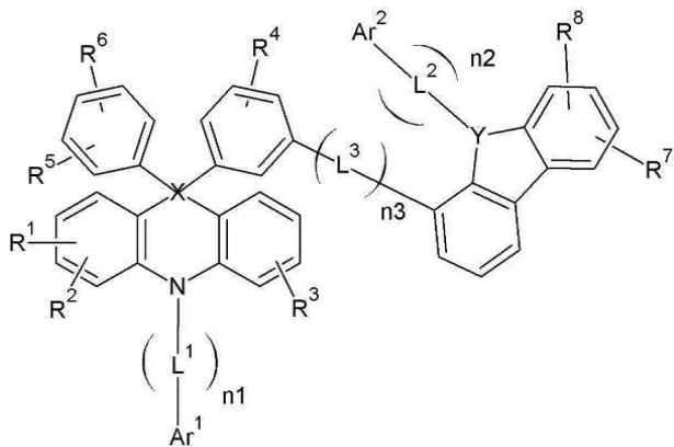
[화학식 1-4]
