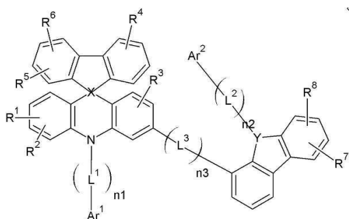
[화학식 4-3]
