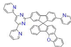
[화학식 B-112]
