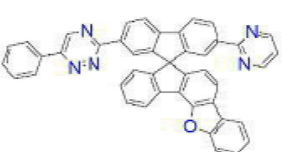
[화학식 B-71]
