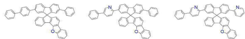
[화학식 B-58] [화학식 B-59] [화학식 B-60]
