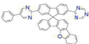
[화학식 B-69]
