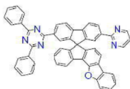
[화학식 B-116]
