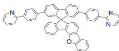
[화학식 B-91]
