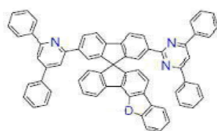
[화학식 B-123]
