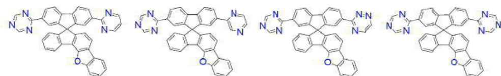
[화학식 B-45] [화학식 B-46] [화학식 B-47] [화학식 B-48]
