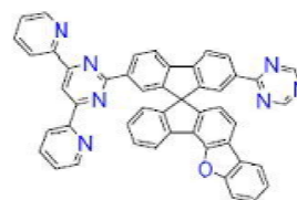
[화학식 B-114]
