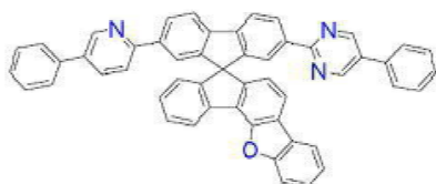
[화학식 B-88]
