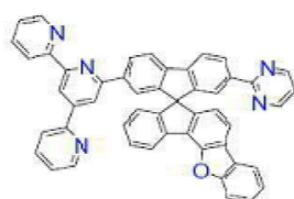
[화학식 B-107]
