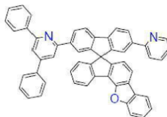
[화학식 B-102]
