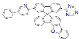
[화학식 B-64]
