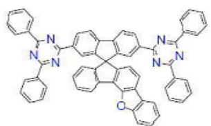
[화학식 B-130]
