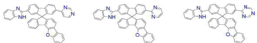
[화학식 B-55] [화학식 B-56] [화학식 B-57]
