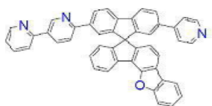
[화학식 B-73]
