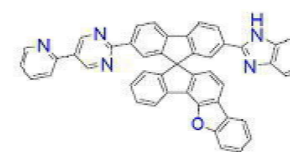
[화학식 B-80]
