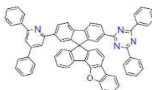
[화학식 B-124]
