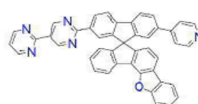
[화학식 B-81]
