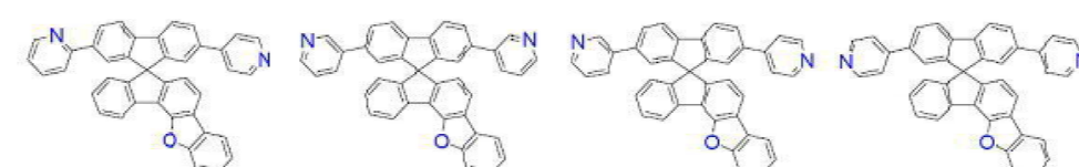
[화학식 B-5]
