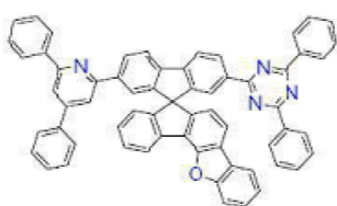
[화학식 B-124]
