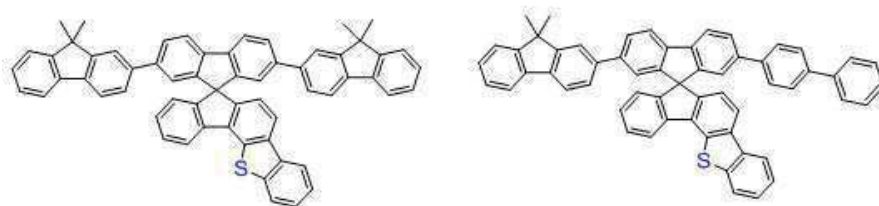
[화학식 A-23]
