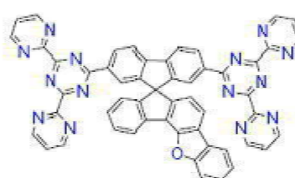
[화학식 B-130]
