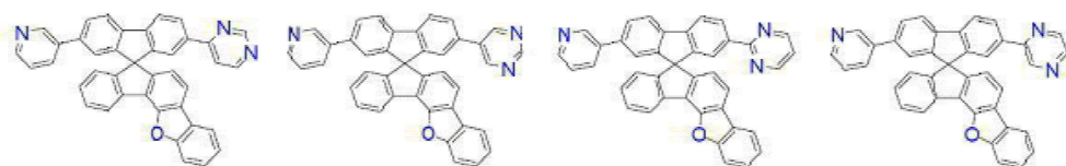
[화학식 B-25] [화학식 B-26] [화학식 B-27] [화학식 B-28]
