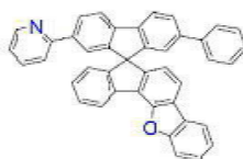
[화학식 B-6]
