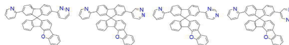
[화학식 B-17]
