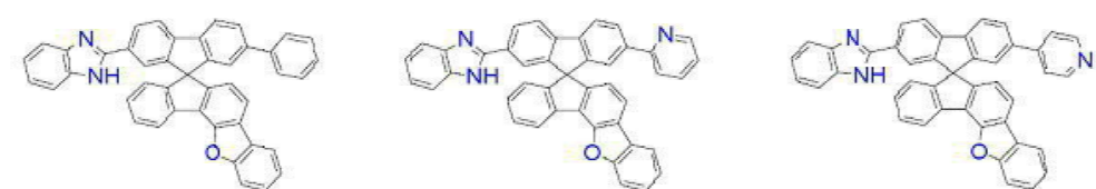
[화학식 B-52] [화학식 B-53] [화학식 B-54]
