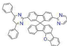
[화학식 B110]
