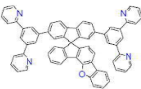
[화학식 B-131]
