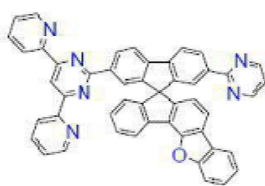
[화학식 B-113]
