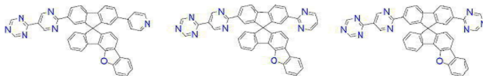
[화학식 B-85]
