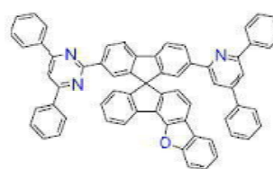
[화학식 B-125]
