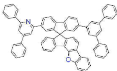
[화학식 B-120]
