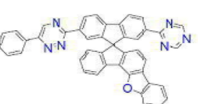
[화학식 B-72]
