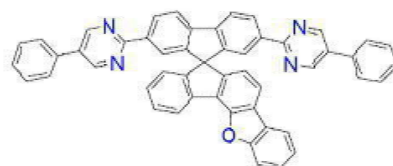
[화학식 B-89]
