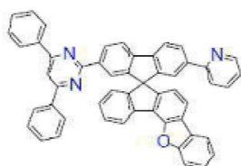
[화학식 B109]
