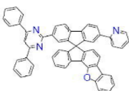
[화학식 B109]
