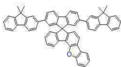
[화학식 A-11]
