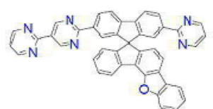
[화학식 B-82]
