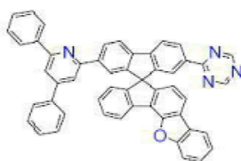
[화학식 B-104]
