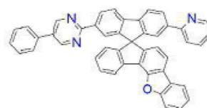
[화학식 B-66]
