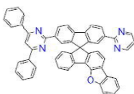
[화학식 B110]
