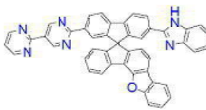
[화학식 B-84]
