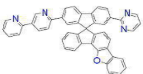
[화학식 B-74]
