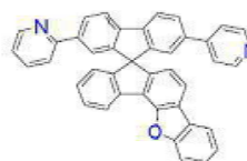
[화학식 B-9]
