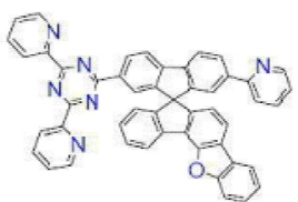
[화학식 B-118]
