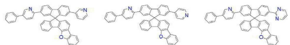
[화학식 B-61] [화학식 B-62] [화학식 B-63]
