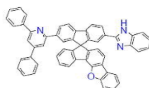
[화학식 B-105]
