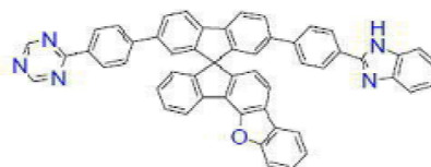
[화학식 B-97]
