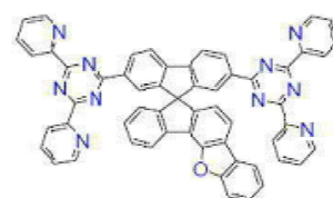
[화학식 B-129]
