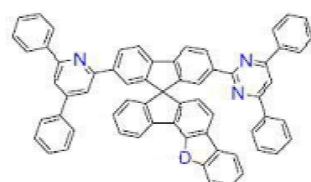
[화학식 B-123]
