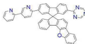
[화학식 B-75]
