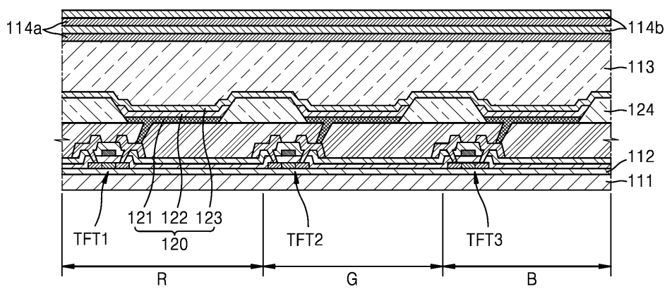
도면4
