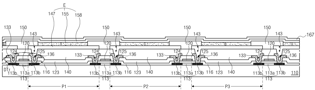
도면5a
