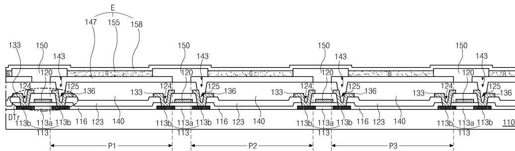
도면4f
