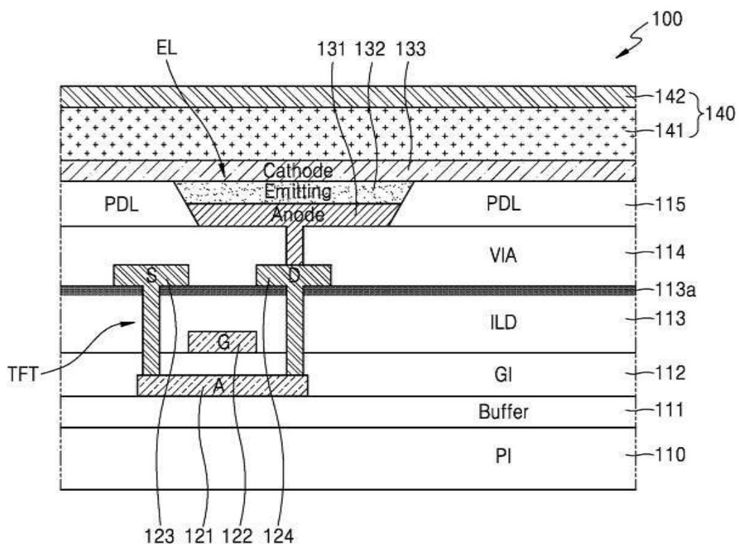
도면4
