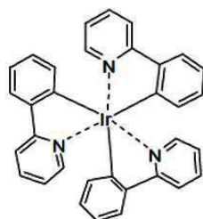
Ir(ppy) 3
