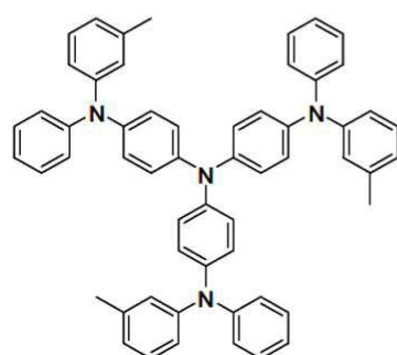
m-MTDATA
