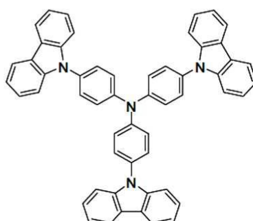
TCTA
