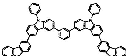
화합물 (H2)
