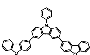
화합물 (H1)
