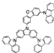
화합물 (15)
