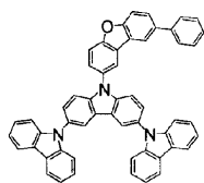
화합물 (2)
