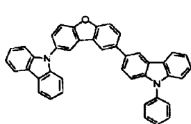
화합물 (H5)
