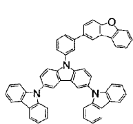
화합물 (32)
