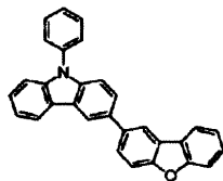
화합물 (H6)
