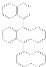
<화합물A>
