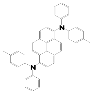
<화합물B>
