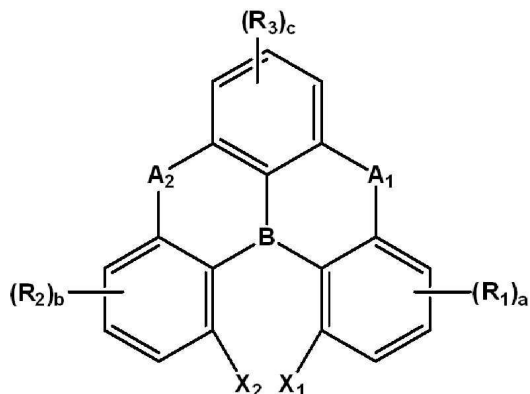
[화학식 1-2]
