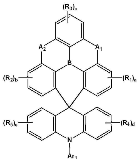
[화학식 3-2]
