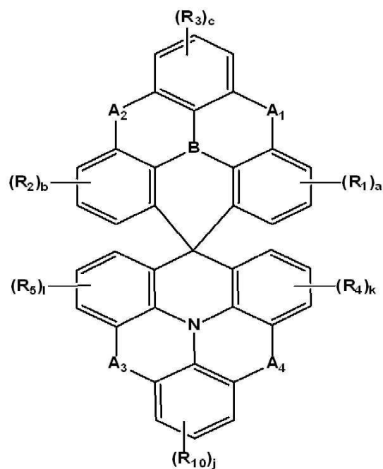
[화학식 3-2]
