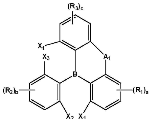
[화학식 1-2]
