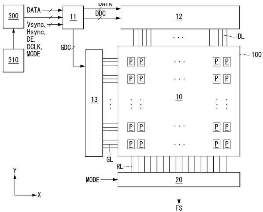
도면3
