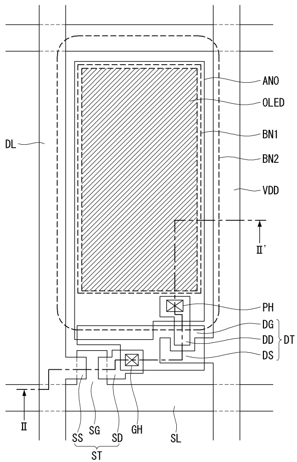
도면6
