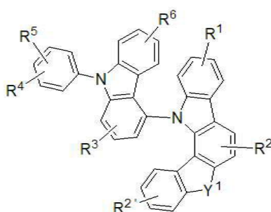
[구조식 4]
