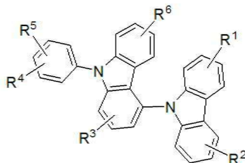
[구조식 2]
