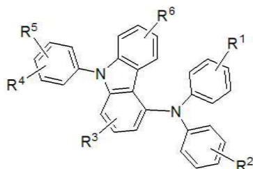
[구조식 1]
