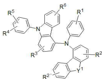
[구조식 3]
