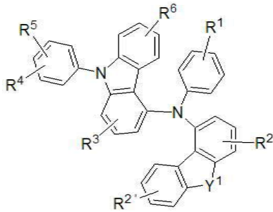
[구조식 3]
