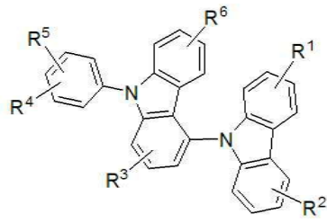
[구조식 2]
