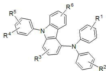
[구조식 1]
