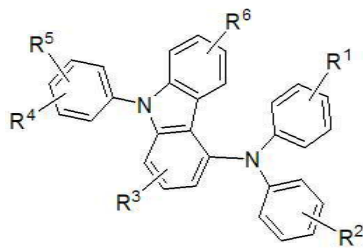
[구조식 1]
