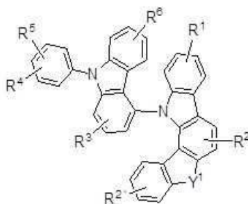
[구조식 4]
