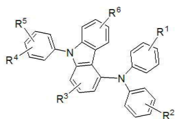
[구조식 1]
