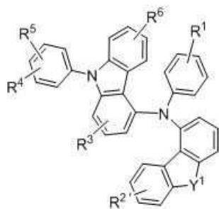
[구조식 3]
