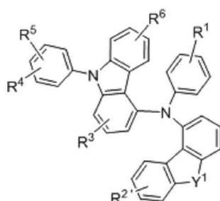
[구조식 3]
