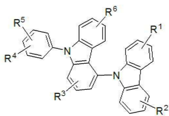
[구조식 2]
