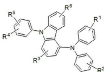
[구조식 1]
