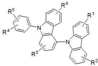
[구조식 2]
