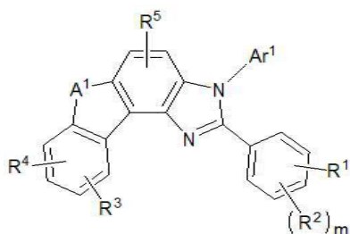
[구조식 2]
