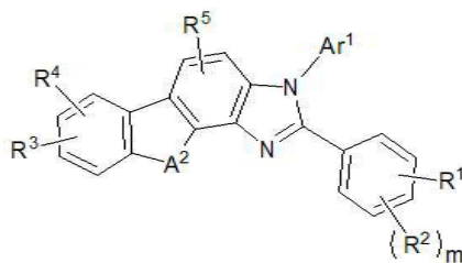
[구조식 3]
