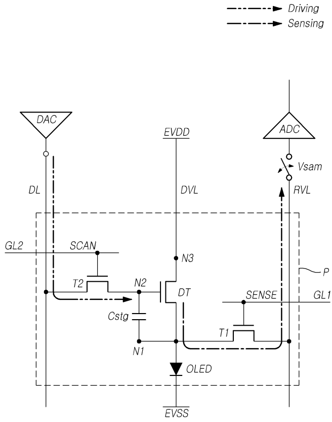
도면2
