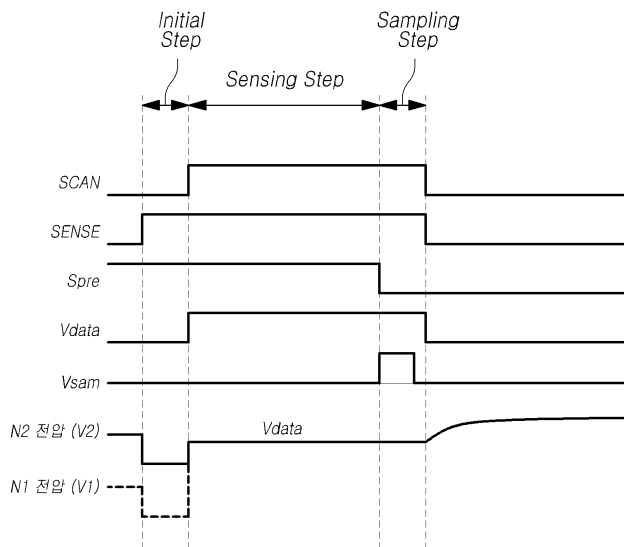
도면22
