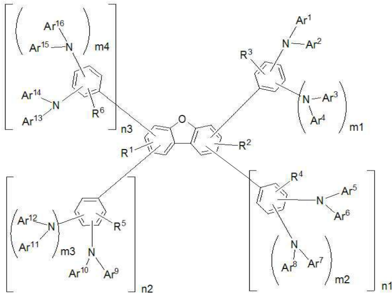
[구조식 1]
