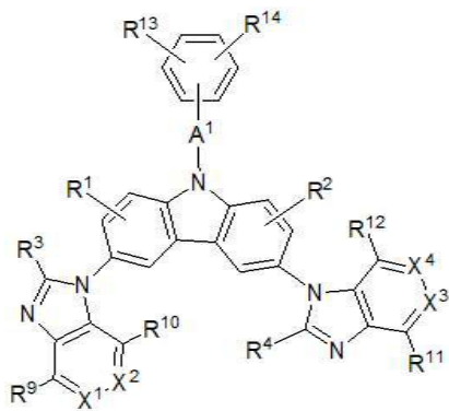
[구조식 4]
