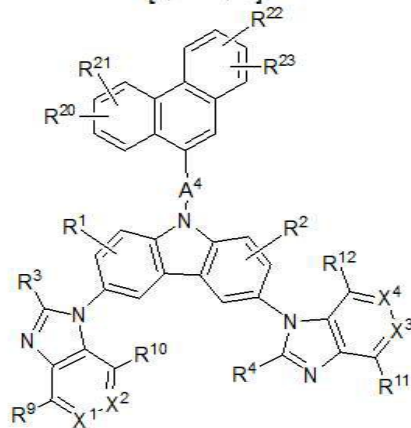
[구조식 5]
