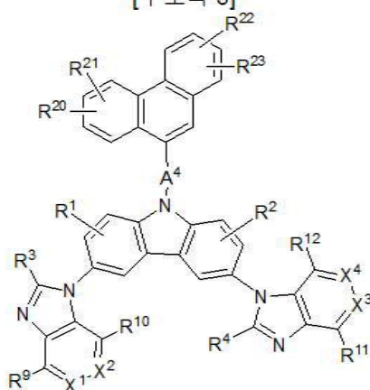
[구조식 7]
