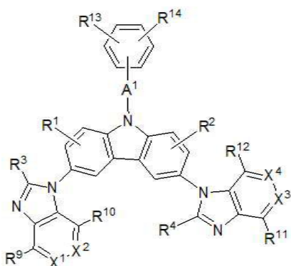
[구조식 2]
