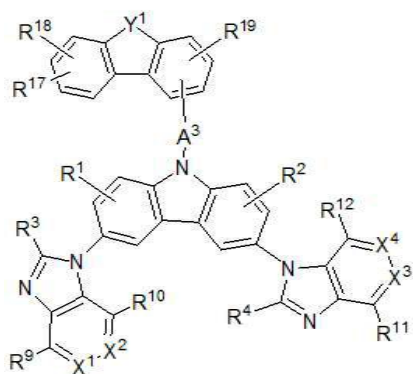
[구조식 6]
