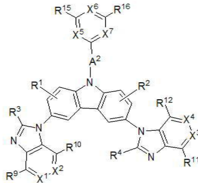
[구조식 3]
