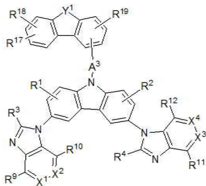
[구조식 6]
