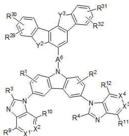
[구조식 7]
