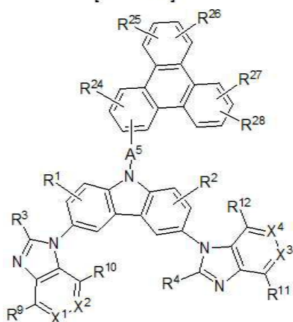
[구조식 6]
