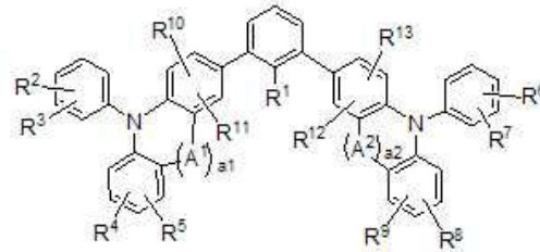
[구조식 4]
