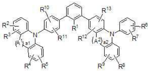
[구조식 1]
