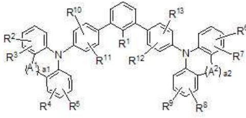
[구조식 2]
