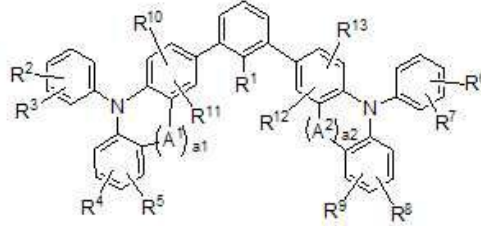
[구조식 4]
