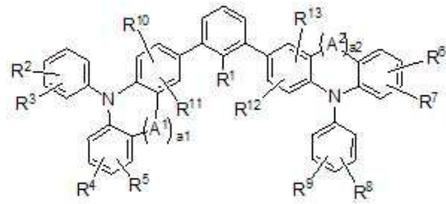
[구조식 5]
