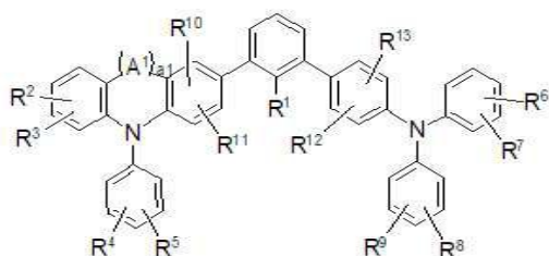
[구조식 9]
