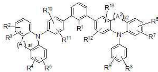
[구조식 3]
