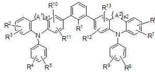
[구조식 6]
