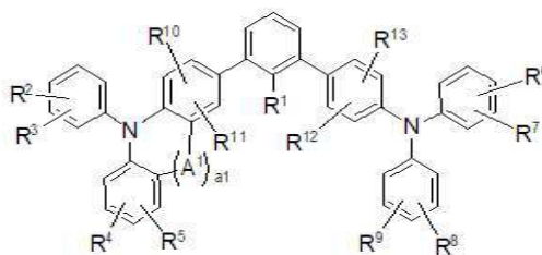
[구조식 8]
