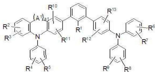
[구조식 9]
