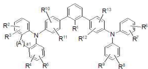
[구조식 9]
