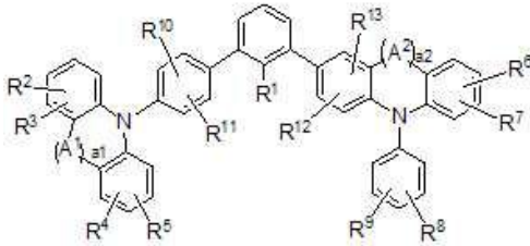
[구조식 3]
