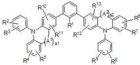
[구조식 5]
