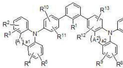
[구조식 3]
