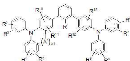
[구조식 8]
