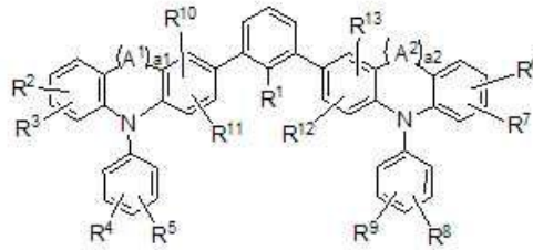
[구조식 6]
