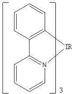
<화학식 c>
