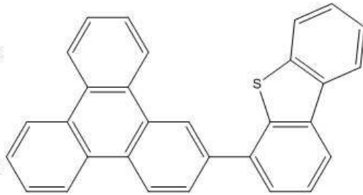
<화학식 b>
