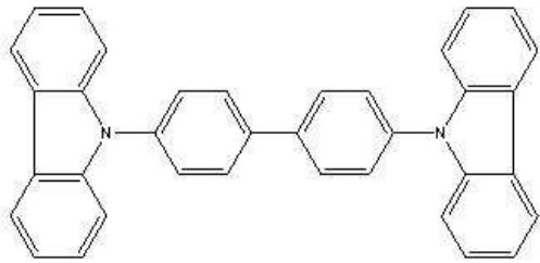
<화학식 c>
