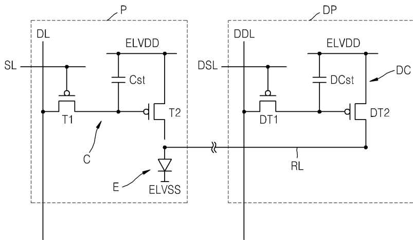
도면16
