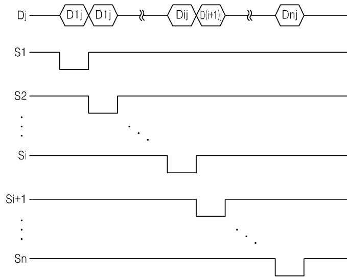
도면12
