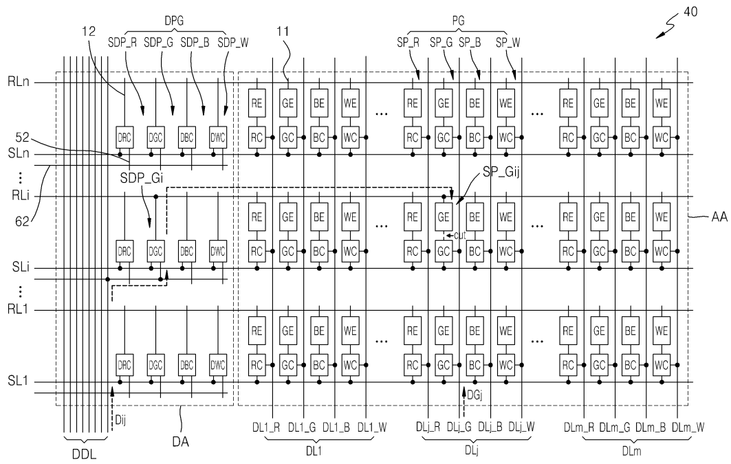
도면14
