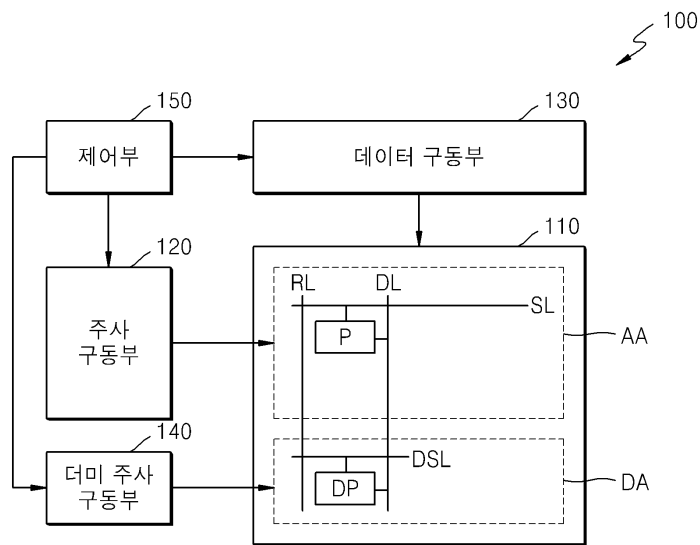
도면1
