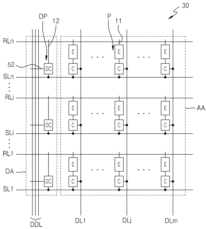
도면10
