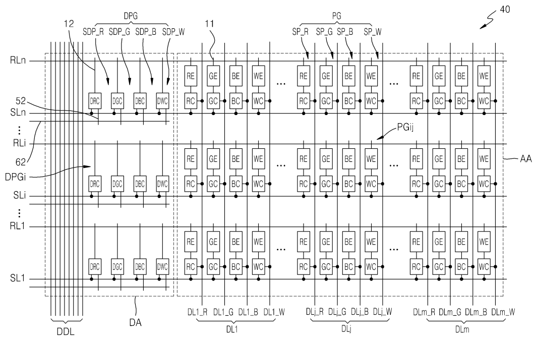
도면12
