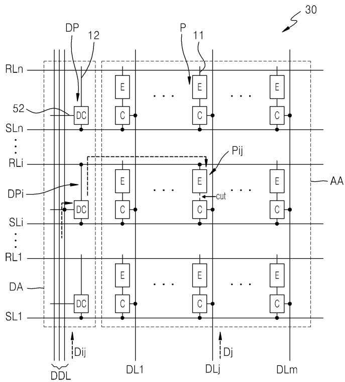
도면10
