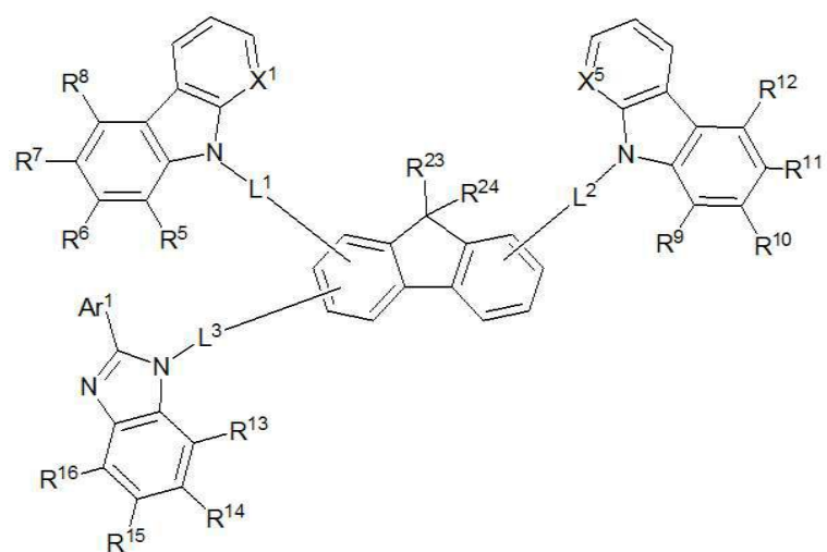
[구조식 6]
