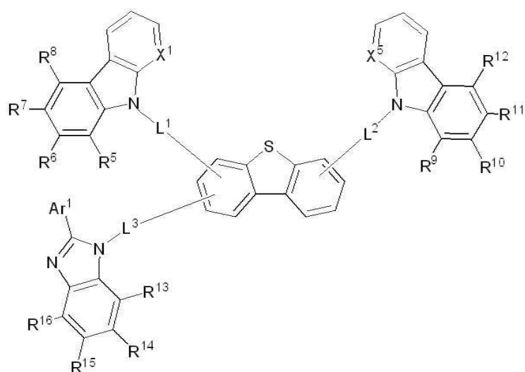
[구조식 5]
