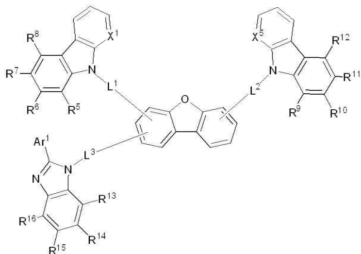
[구조식 4]
