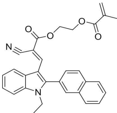
<화학식 1-4>
