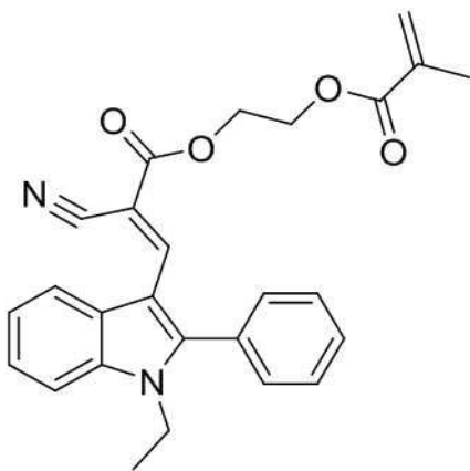
<화학식 1-4>
