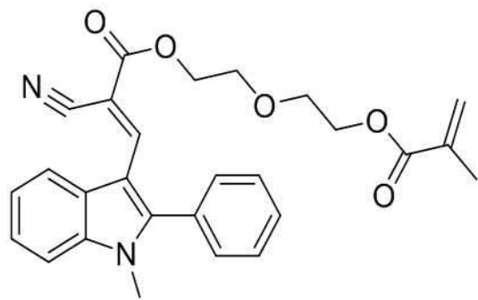
<화학식 1-3>
